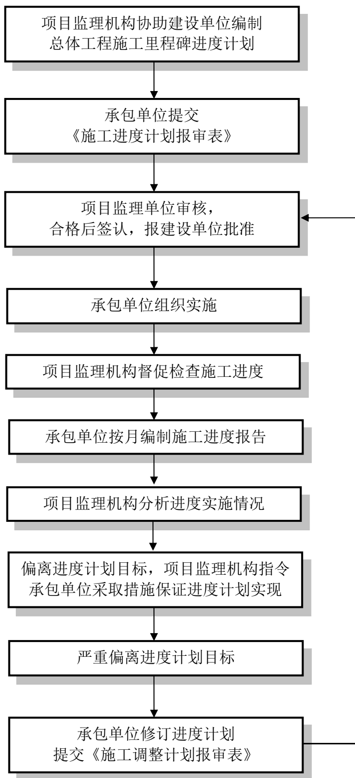
图 B.1 施工阶段工程质量监理程序框图
