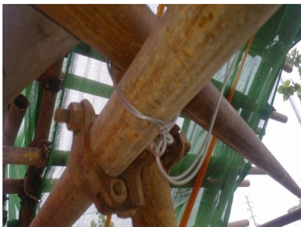
脚手架未用固定件连接，安全等级不够
