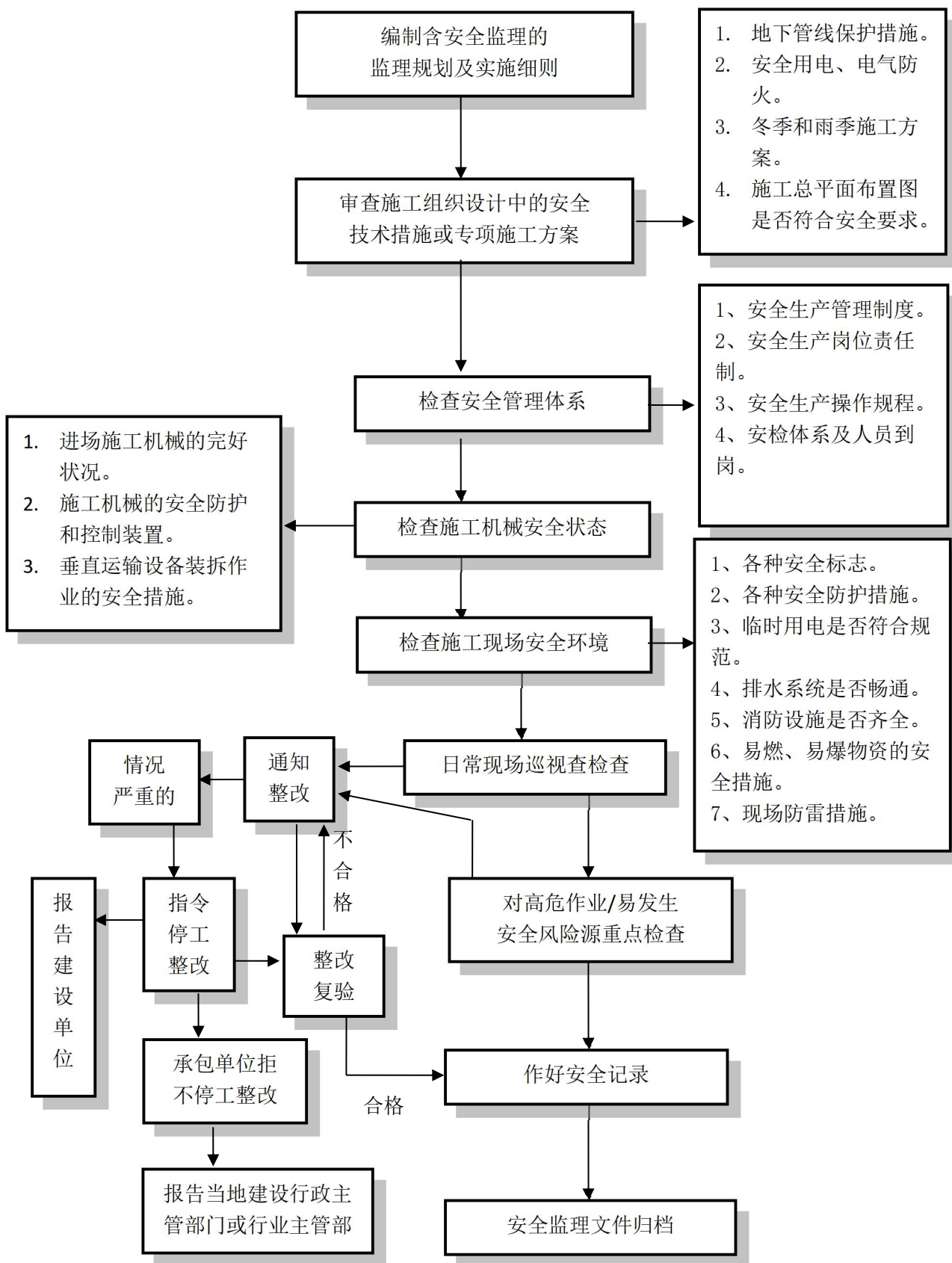
图 4.1 施工阶段工程安全监理程序框图
