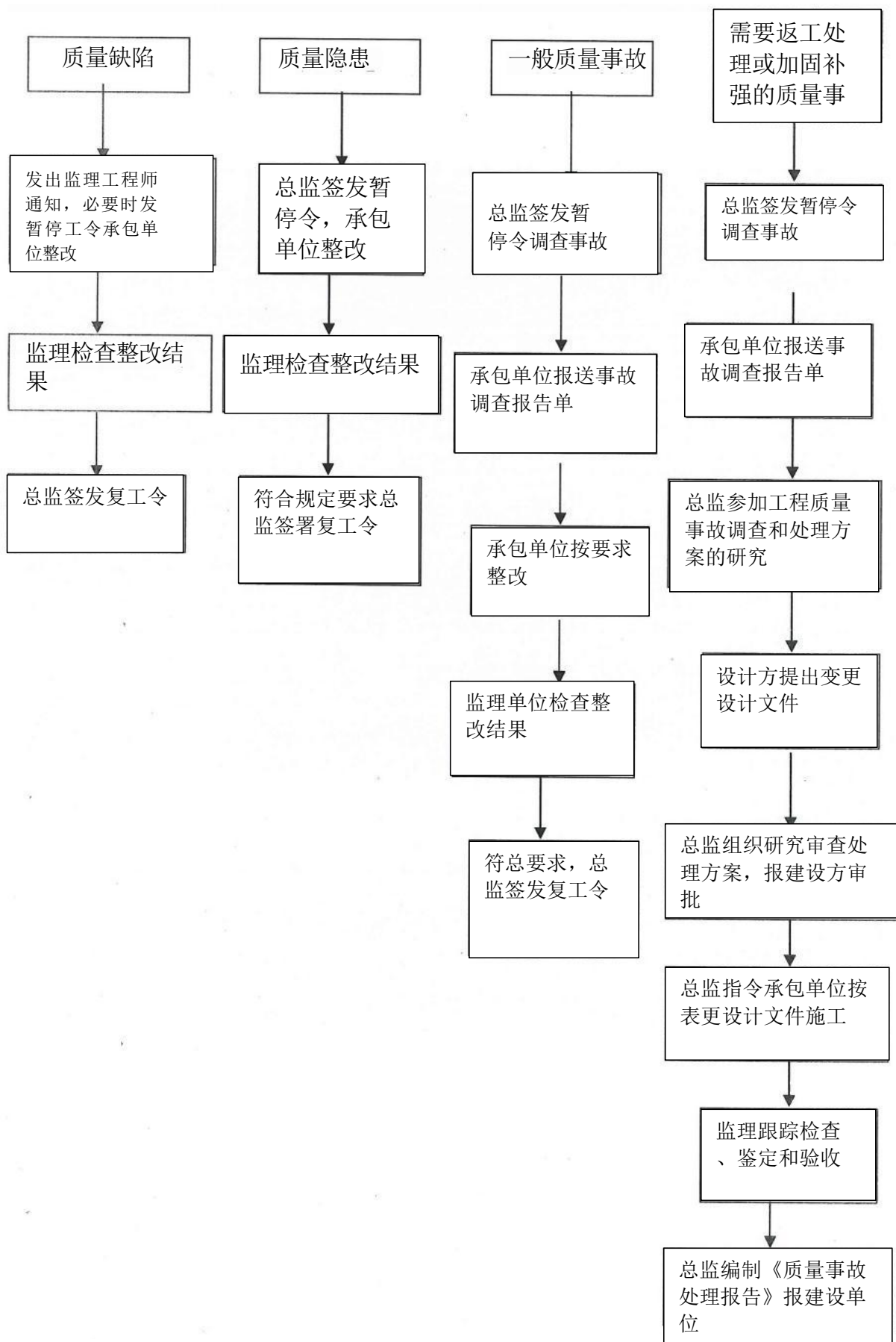
12、工程质量缺陷、质量隐患处理程序框图(框图12)
