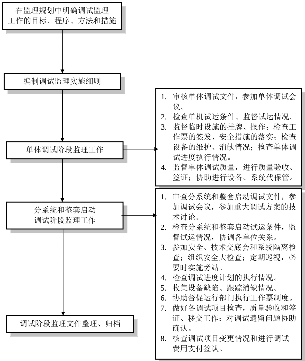
图 B.9 调试阶段监理工作程序框图
