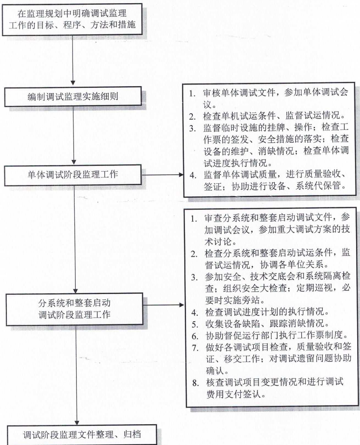
图 B.9 调试阶段监督工作程序框图
