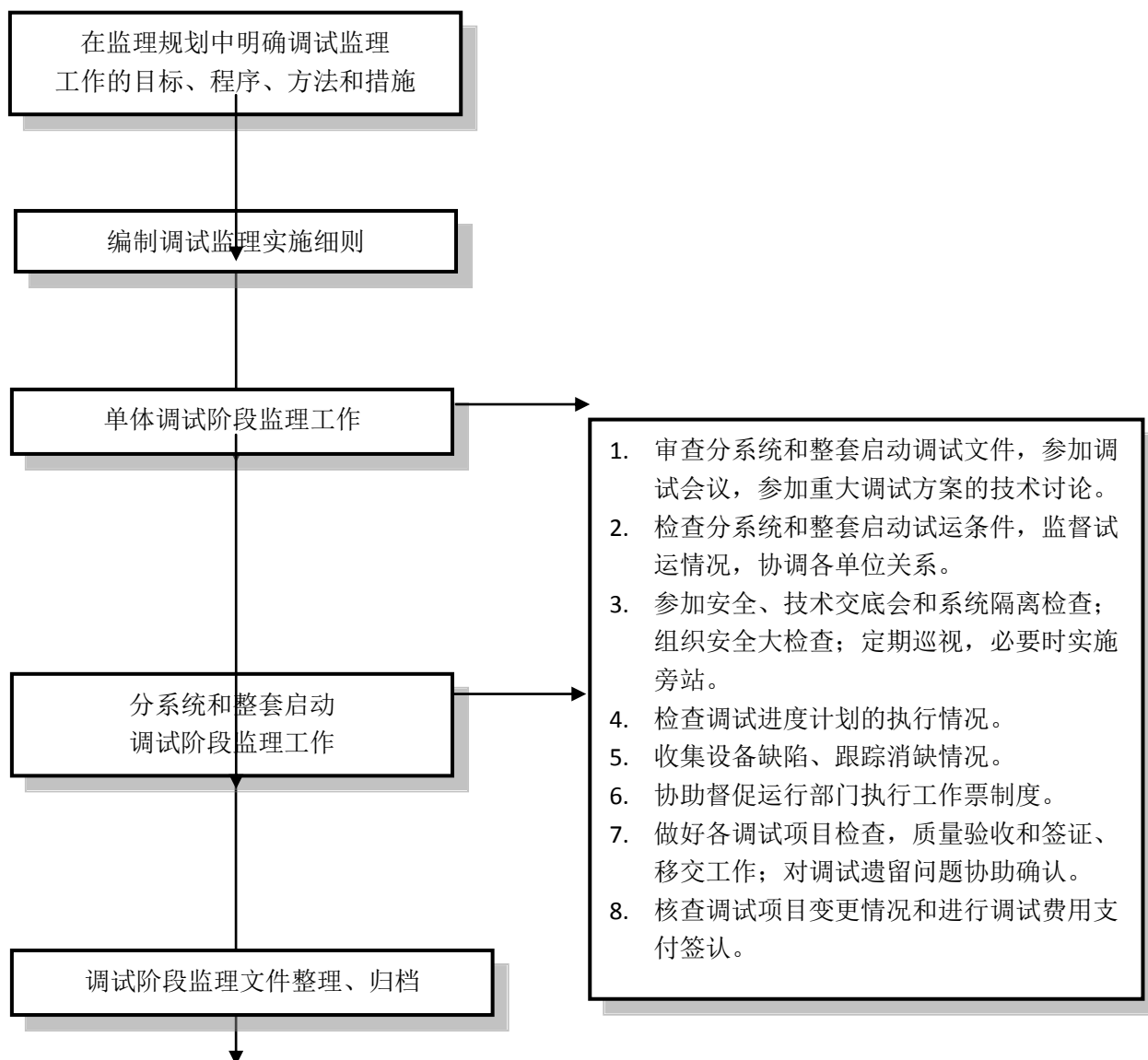
图 B.9 调试阶段监理工作程序框图
