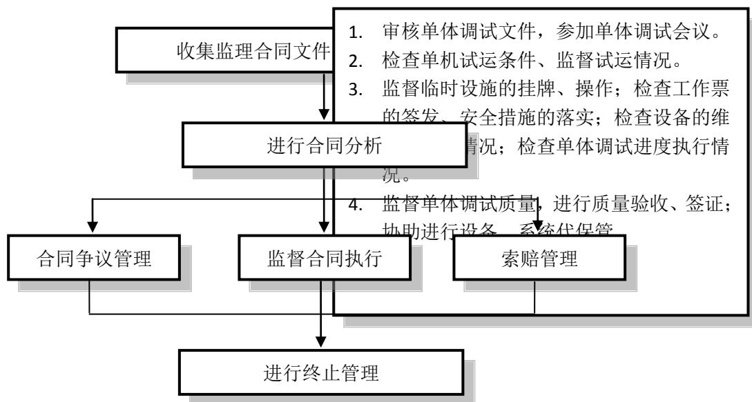
图 B.5 施工阶段工程合同管理程序框图
