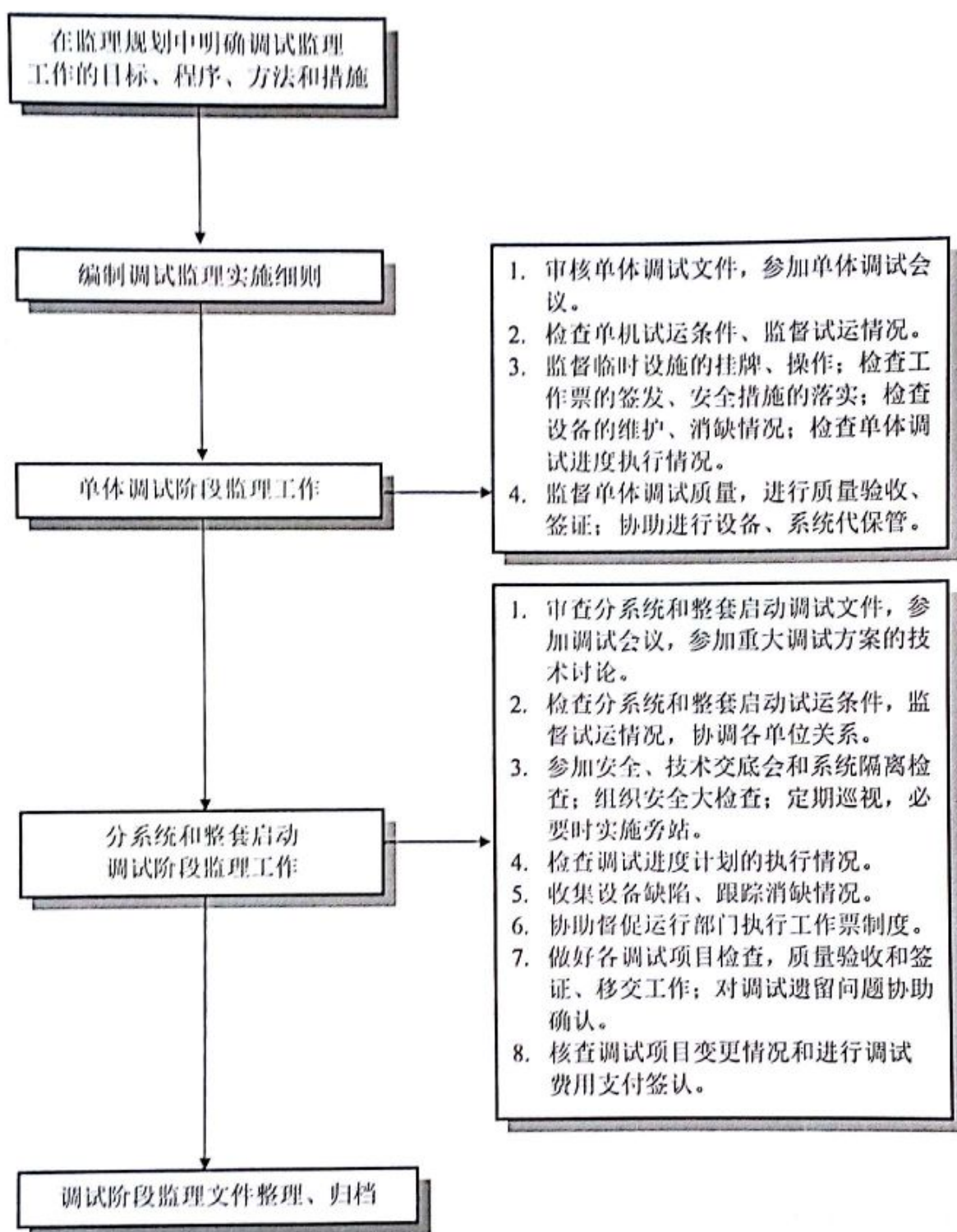
图 B.9 调试阶段监理工作程序框图
