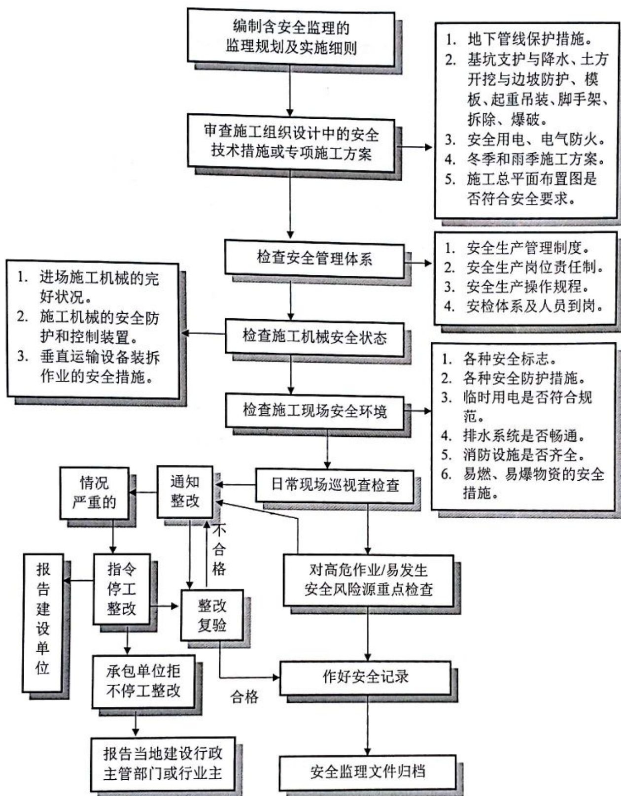
图 B.4 施工阶段工程安全监督程序框图
