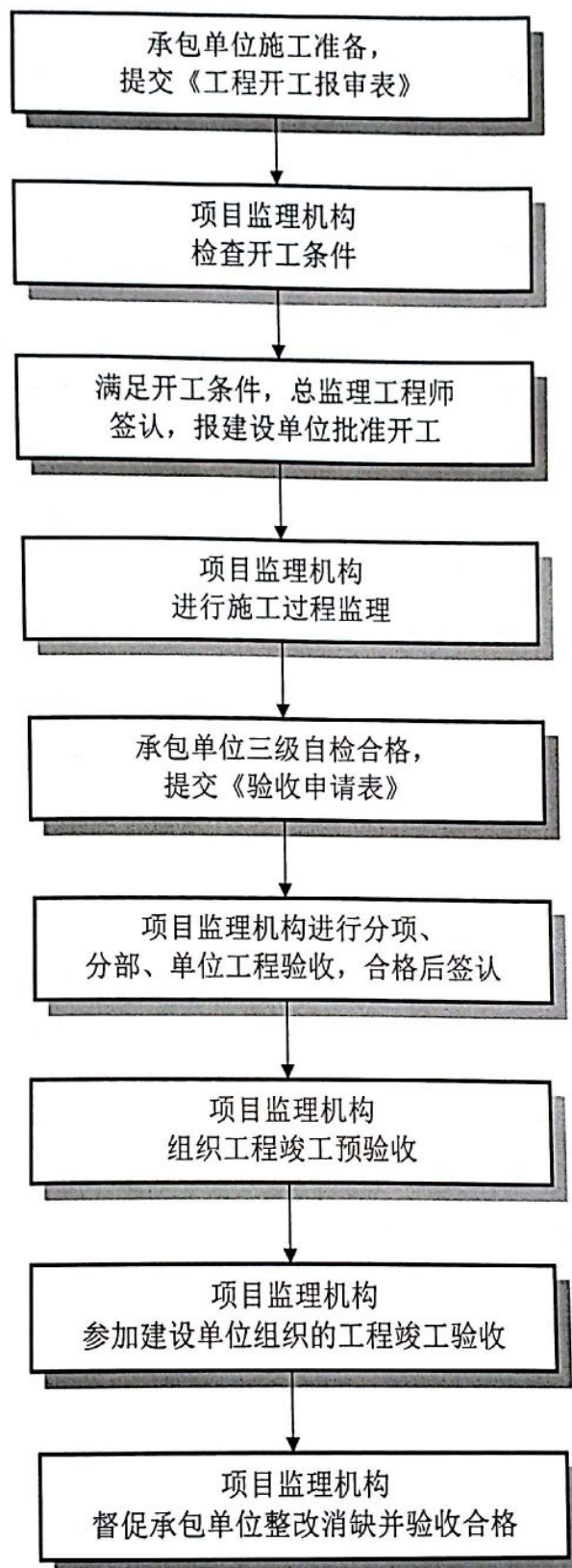
图 2.1 施工阶段工程质量和安全监理程序图
