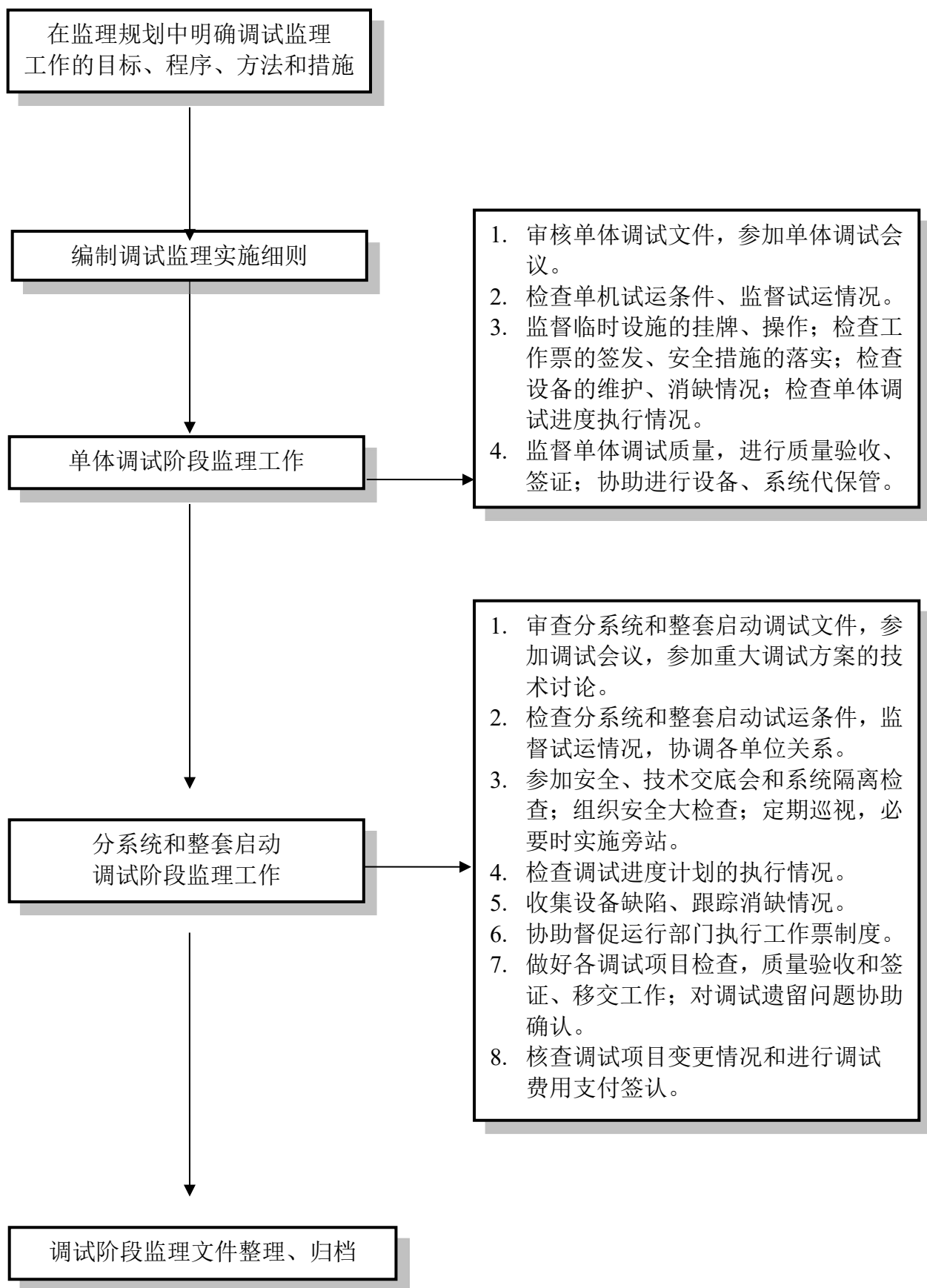
图 B.6 调试阶段监理工作程序框图
