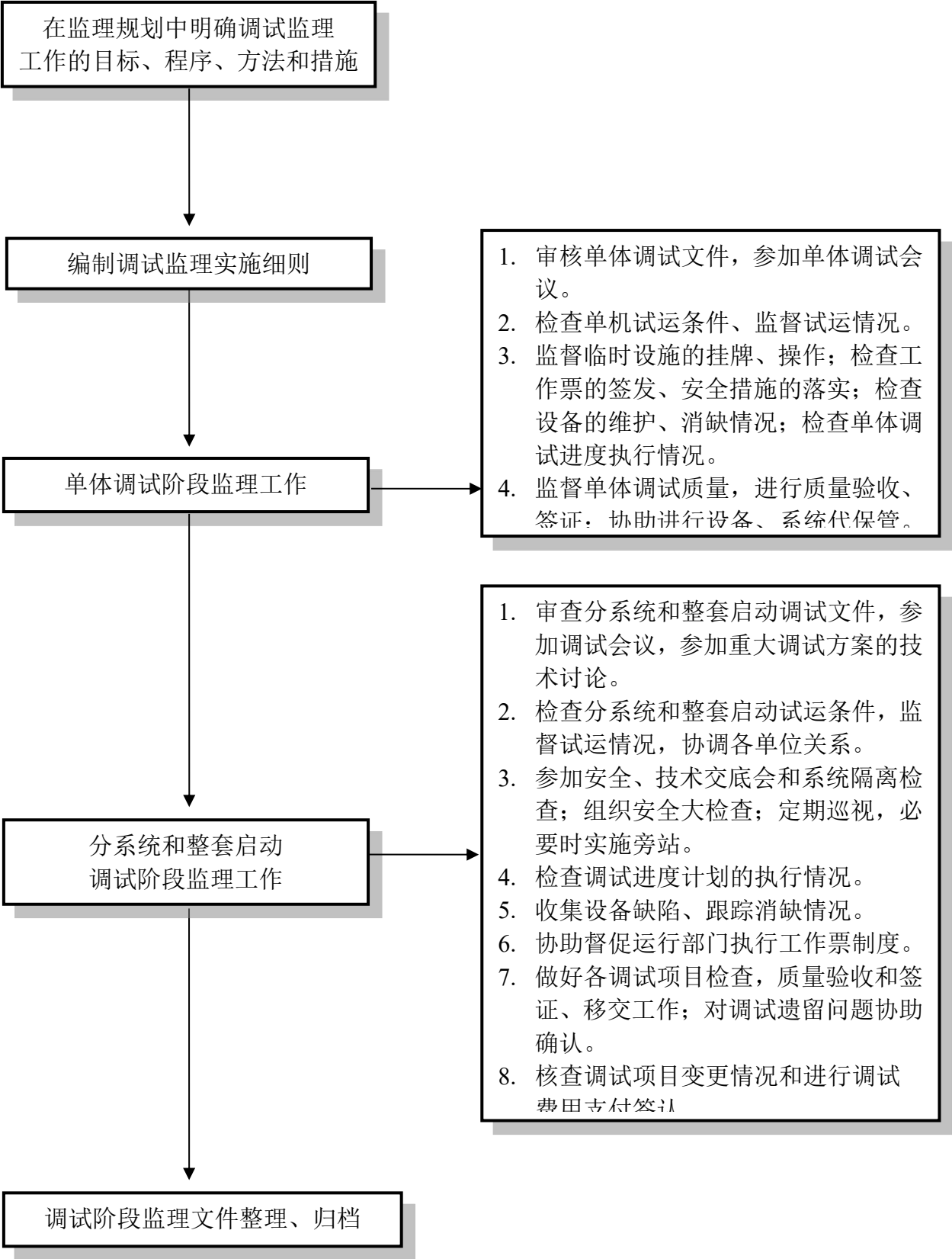
图 B.9 调试阶段监理工作程序框图
