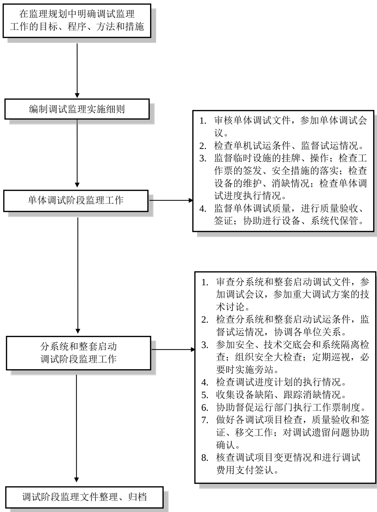
图 B.9 调试阶段监理工作程序框图
