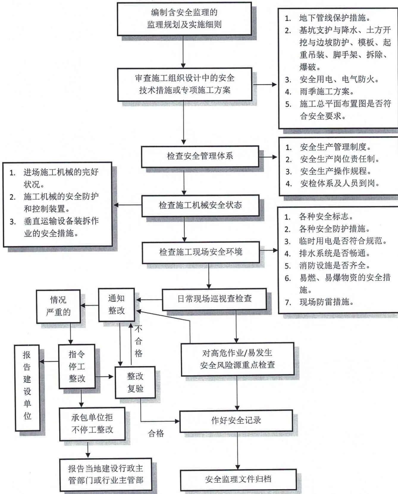
图 B.4 施工阶段工程安全监督程序框图
