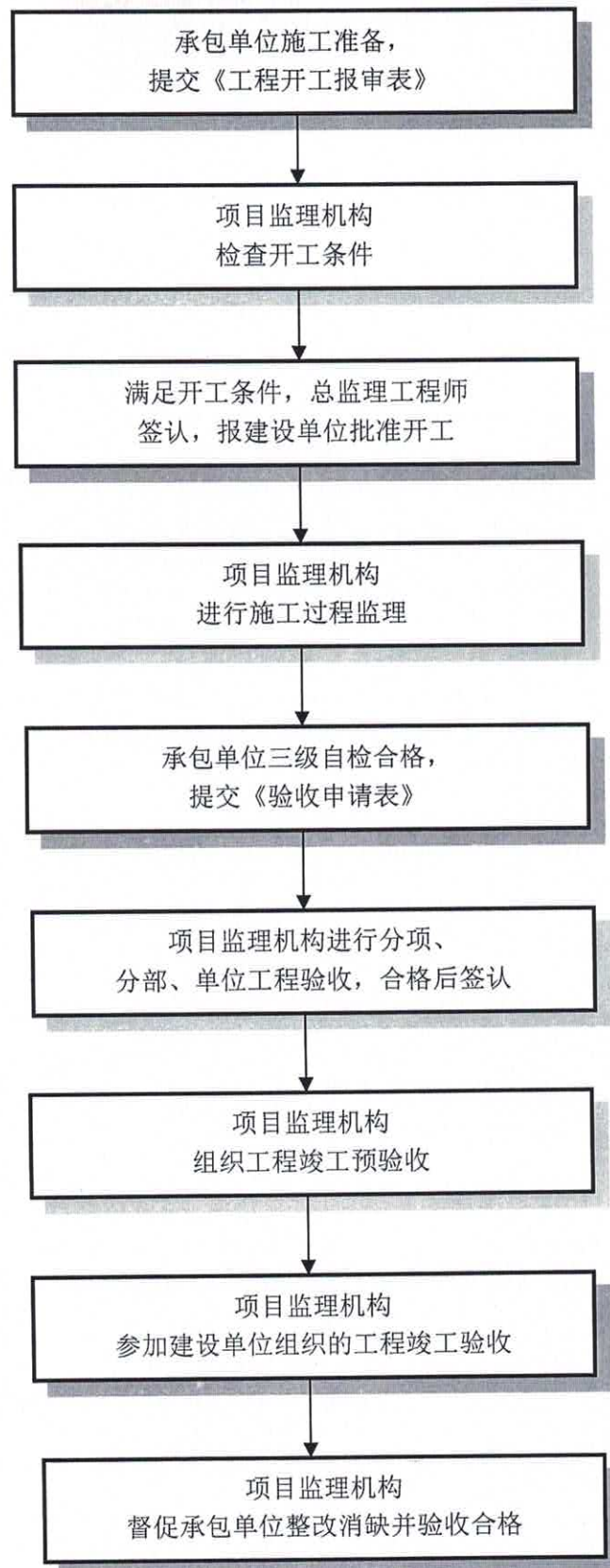
图 B.1 施工阶段工程质量监程序框图
