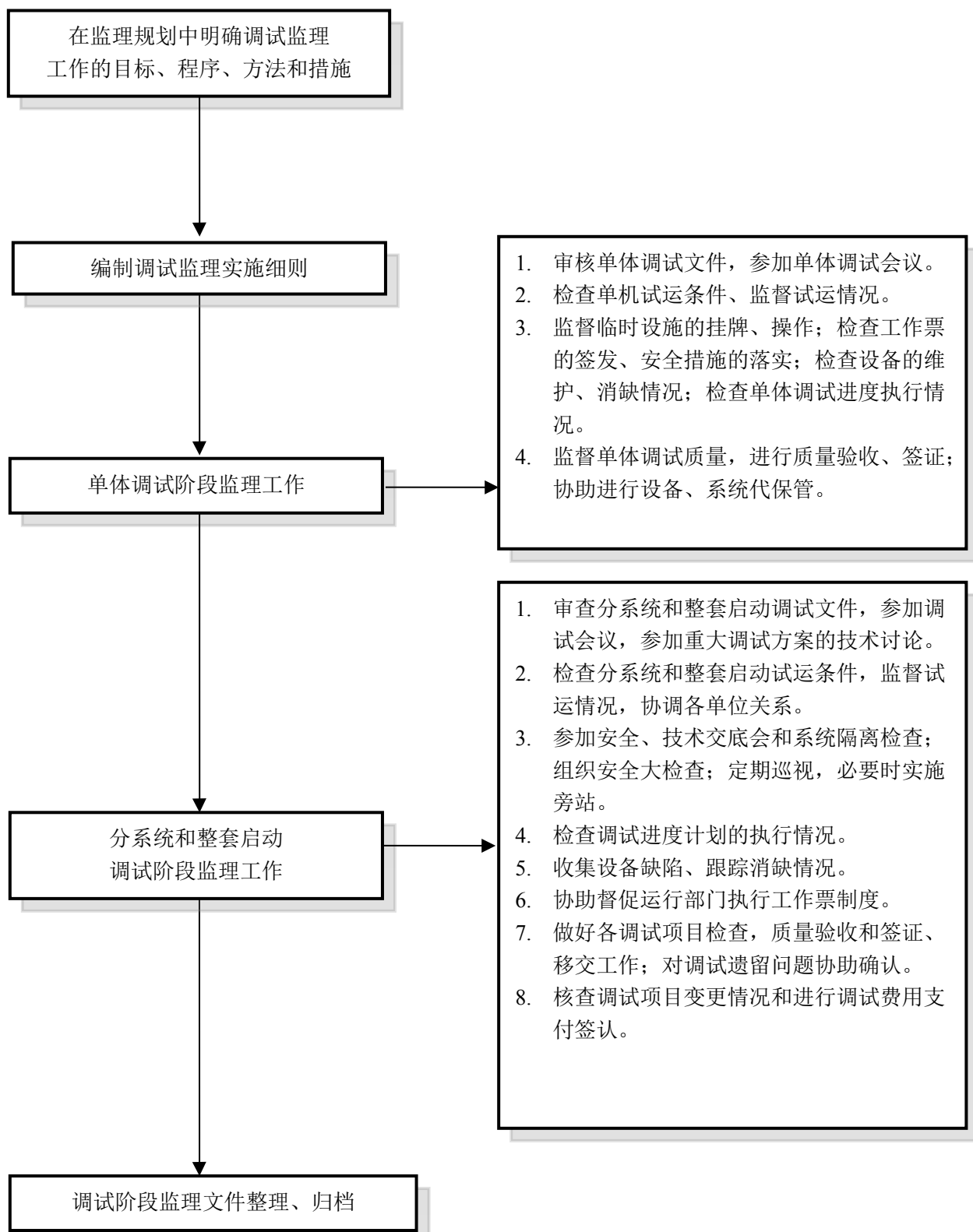
图 B.6 调试阶段监理工作程序框图
