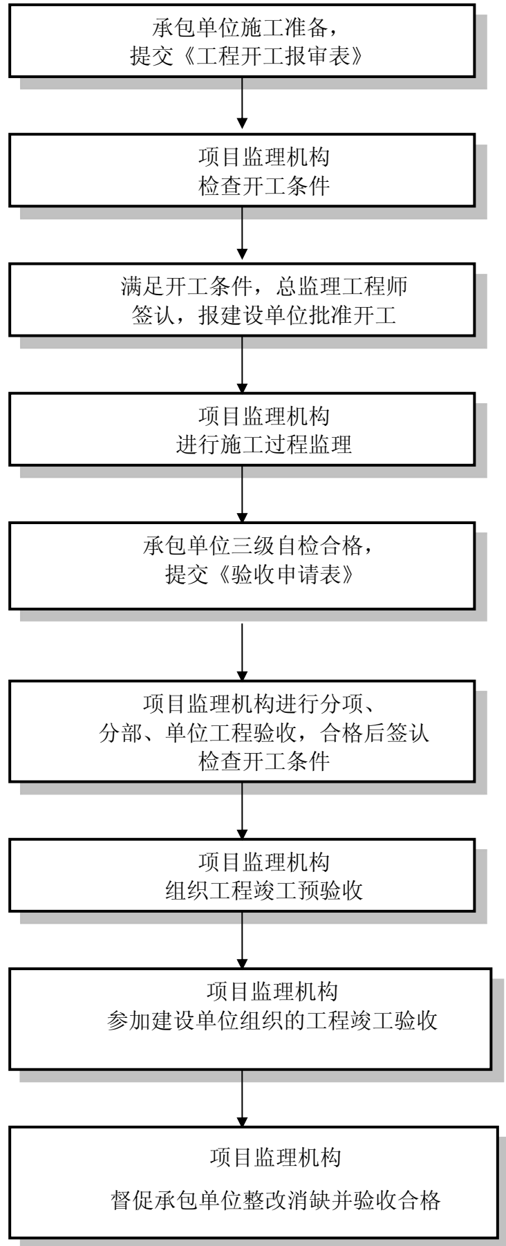
图 B.1 施工阶段工程质量监理程序框图
