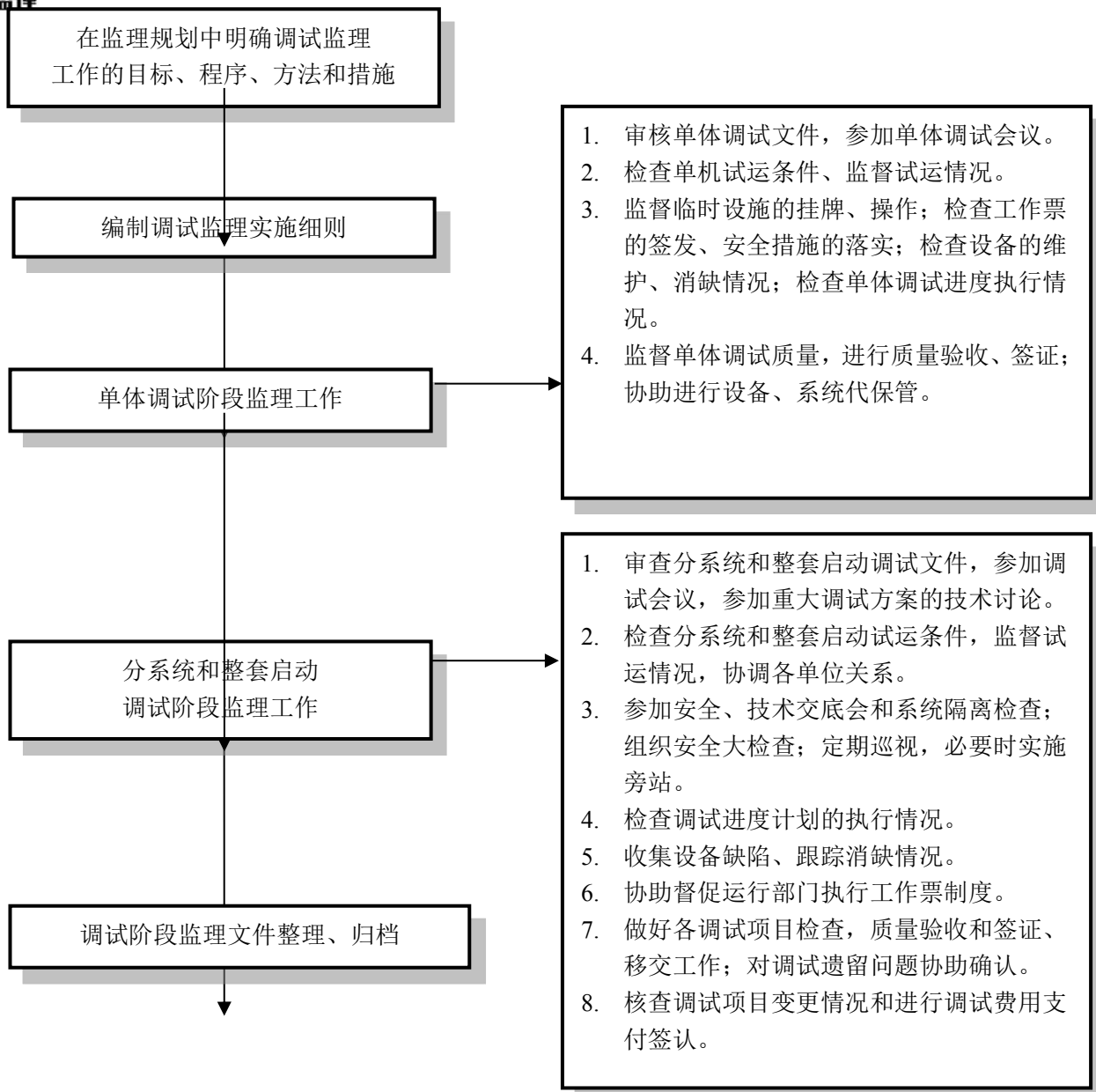
图 B.9 调试阶段监理工作程序框图
