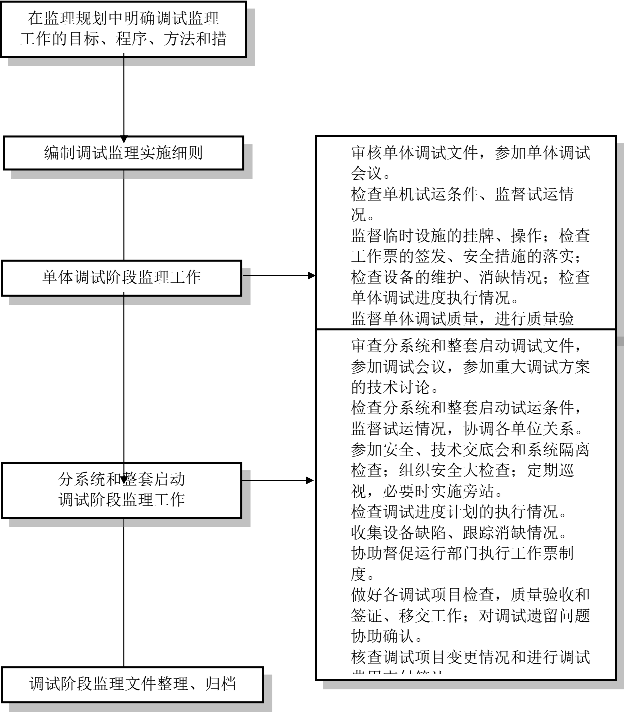
图 B.9 调试阶段监理工作程序框图
