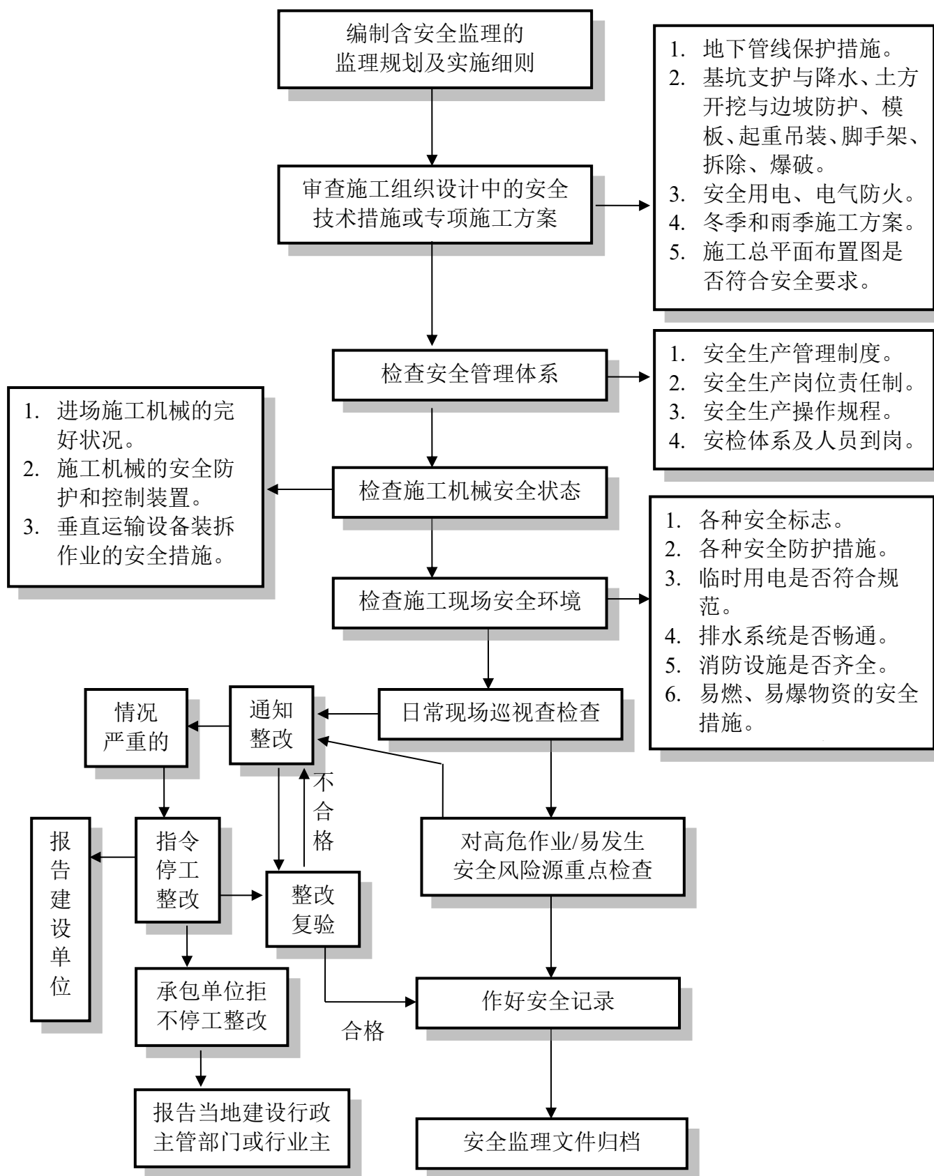
图 B.3 施工阶段工程安全监理程序框图
