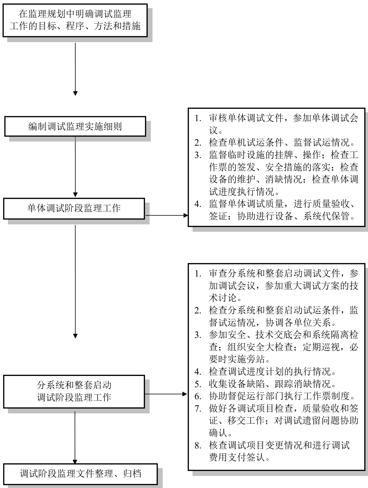
图 B.6 调试阶段监理工作程序框图
