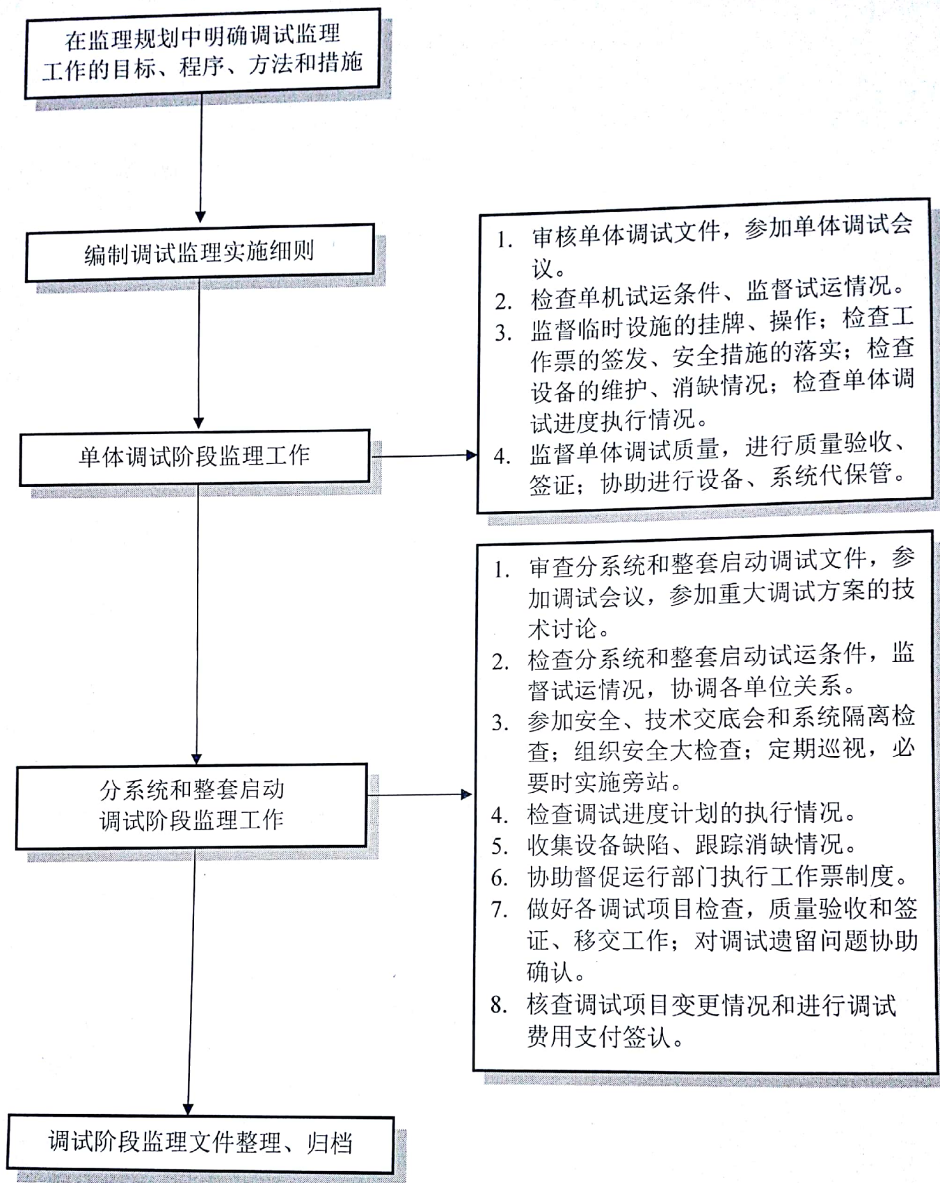
图 B.9 调试阶段监理工作程序框图
