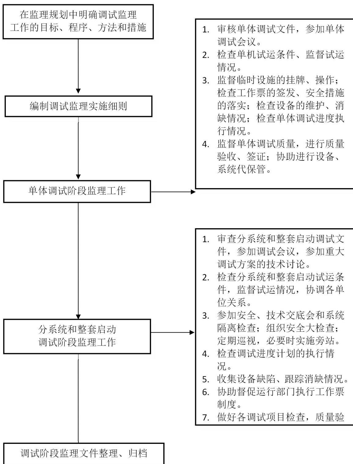
图 B.9 调试阶段监理工作程序框图
