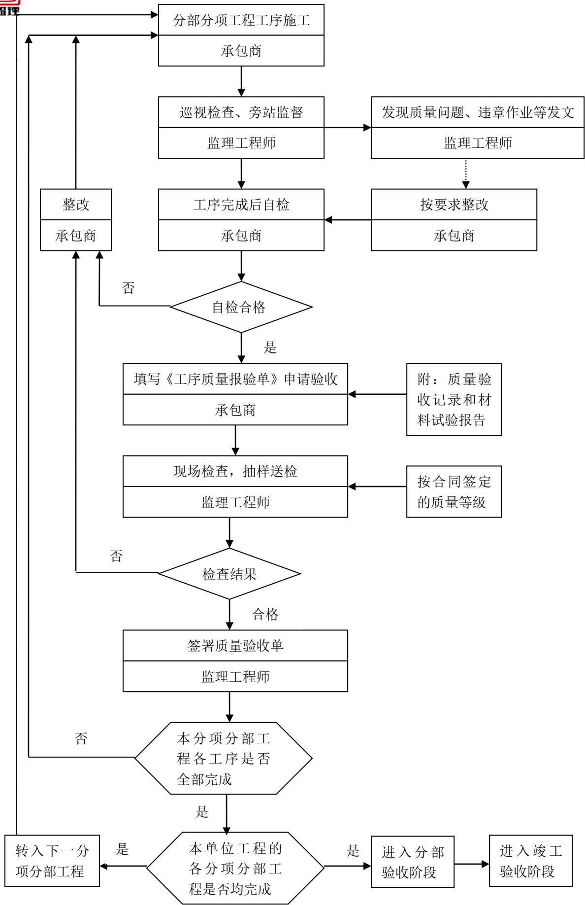
e、施工阶段质量控制工作流程图
