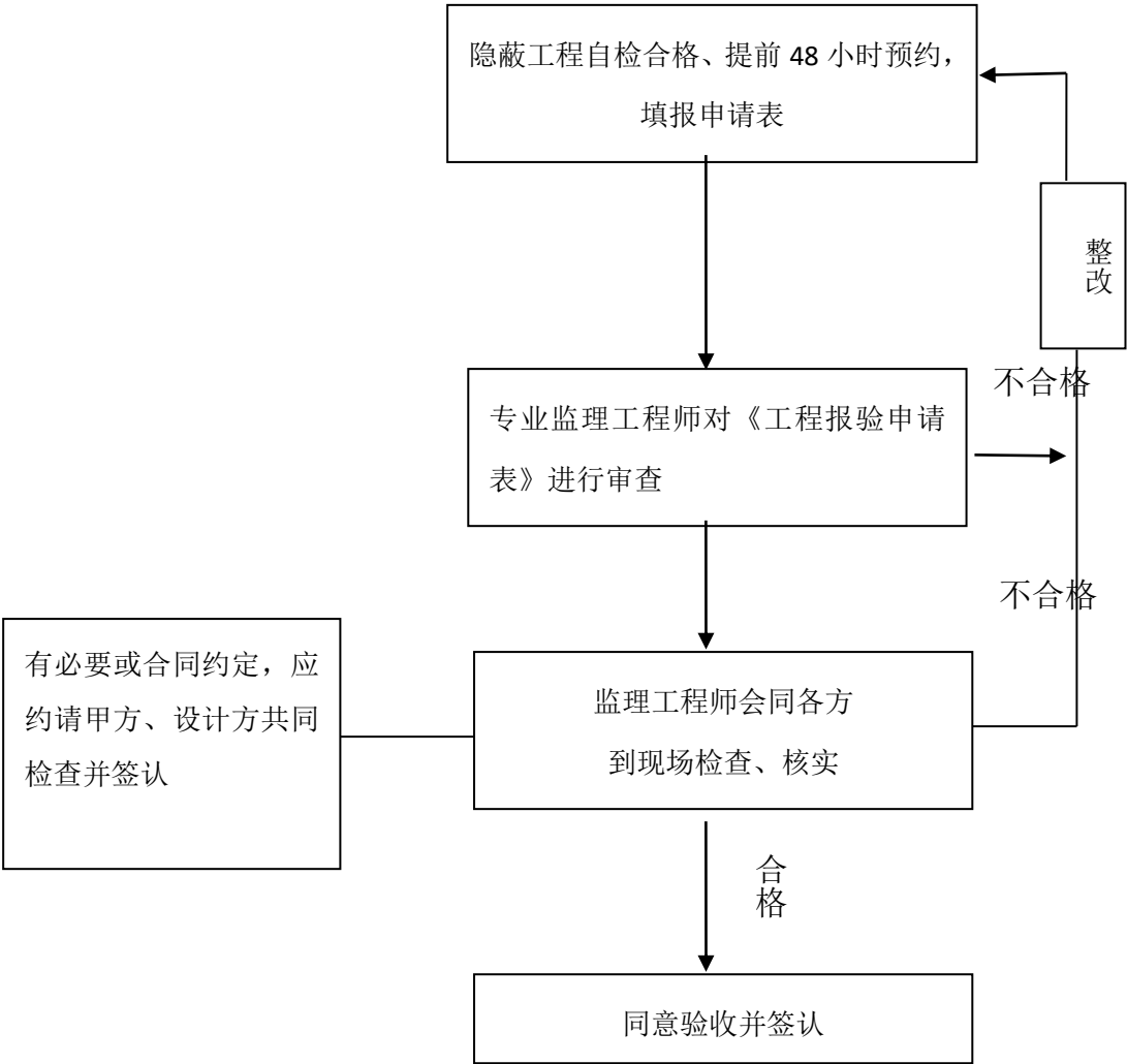
7、隐蔽工程检查验收程序框图（框图 7）
