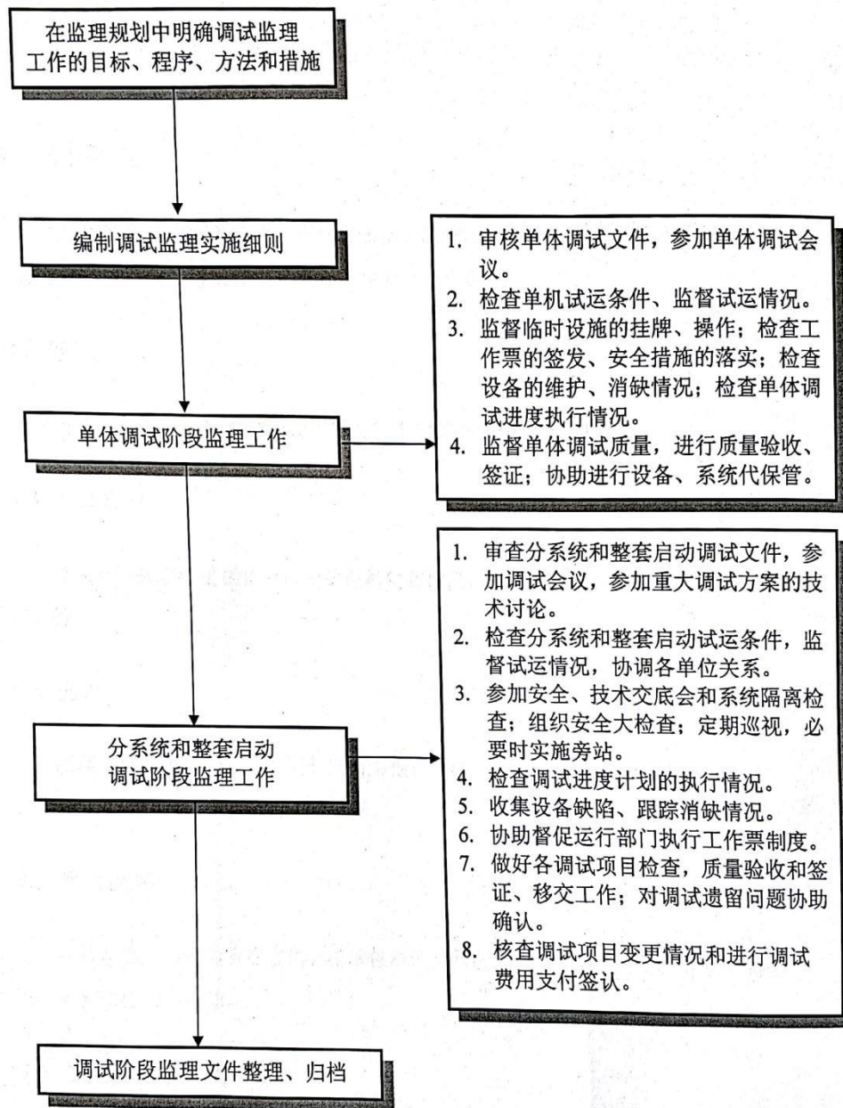
图 B.9 调试阶段监理工作程序框图
