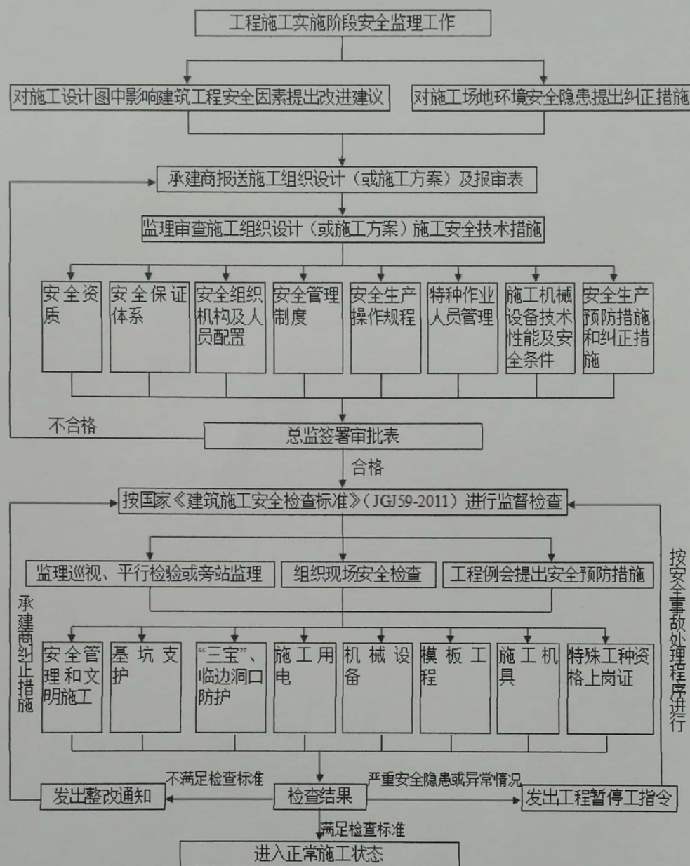
安全生产管理监理工作流程图
