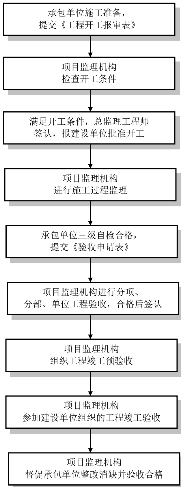
图 B.1 施工阶段 3 工程质量监理程序框图
