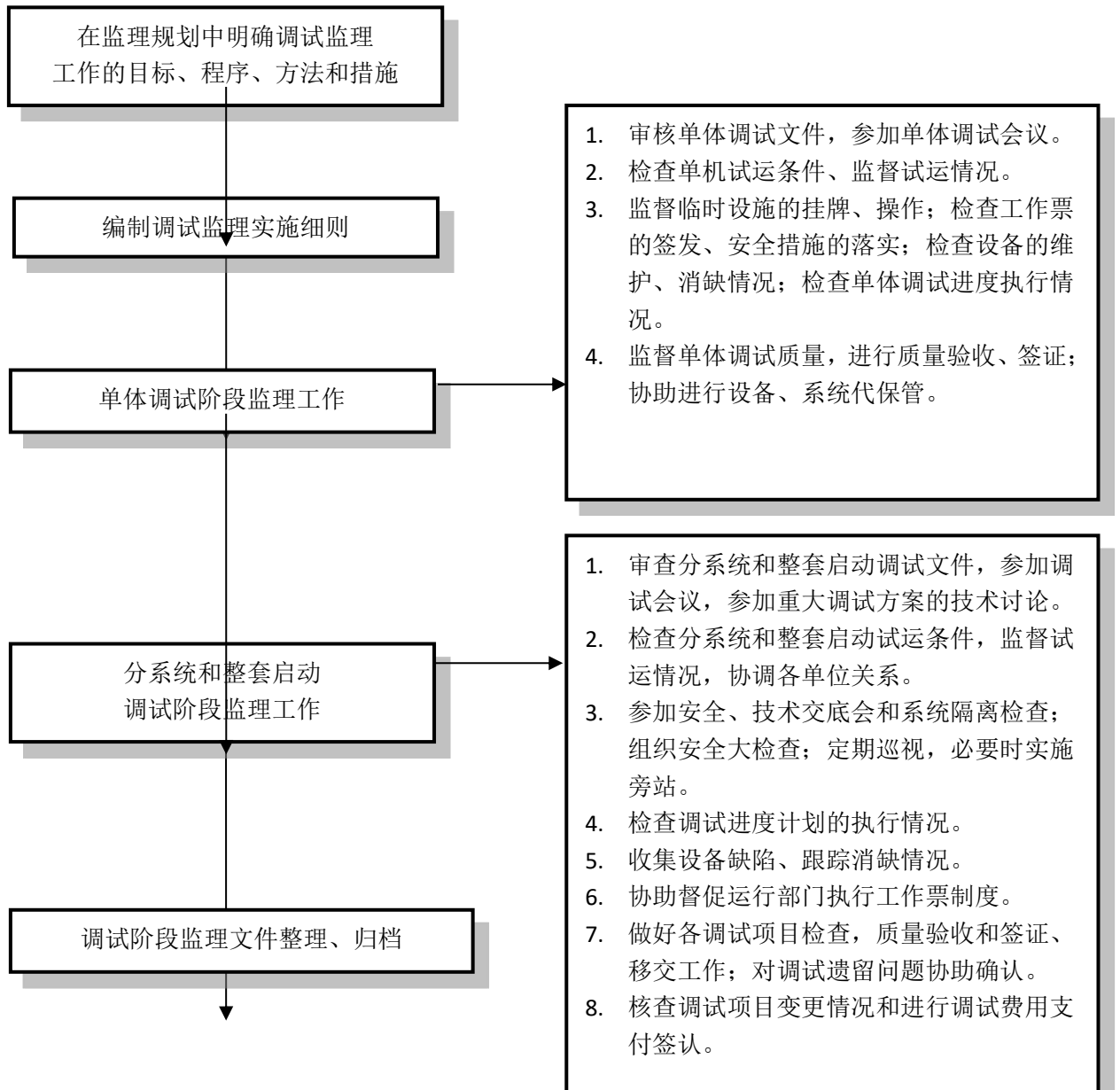
图 B.9 调试阶段监理工作程序框图
