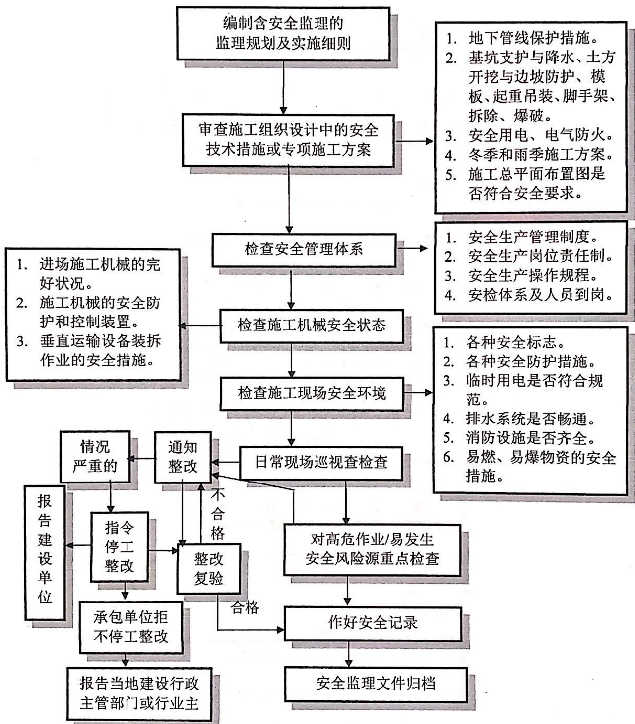
图 B.3 施工阶段工程安全监理程序框图
