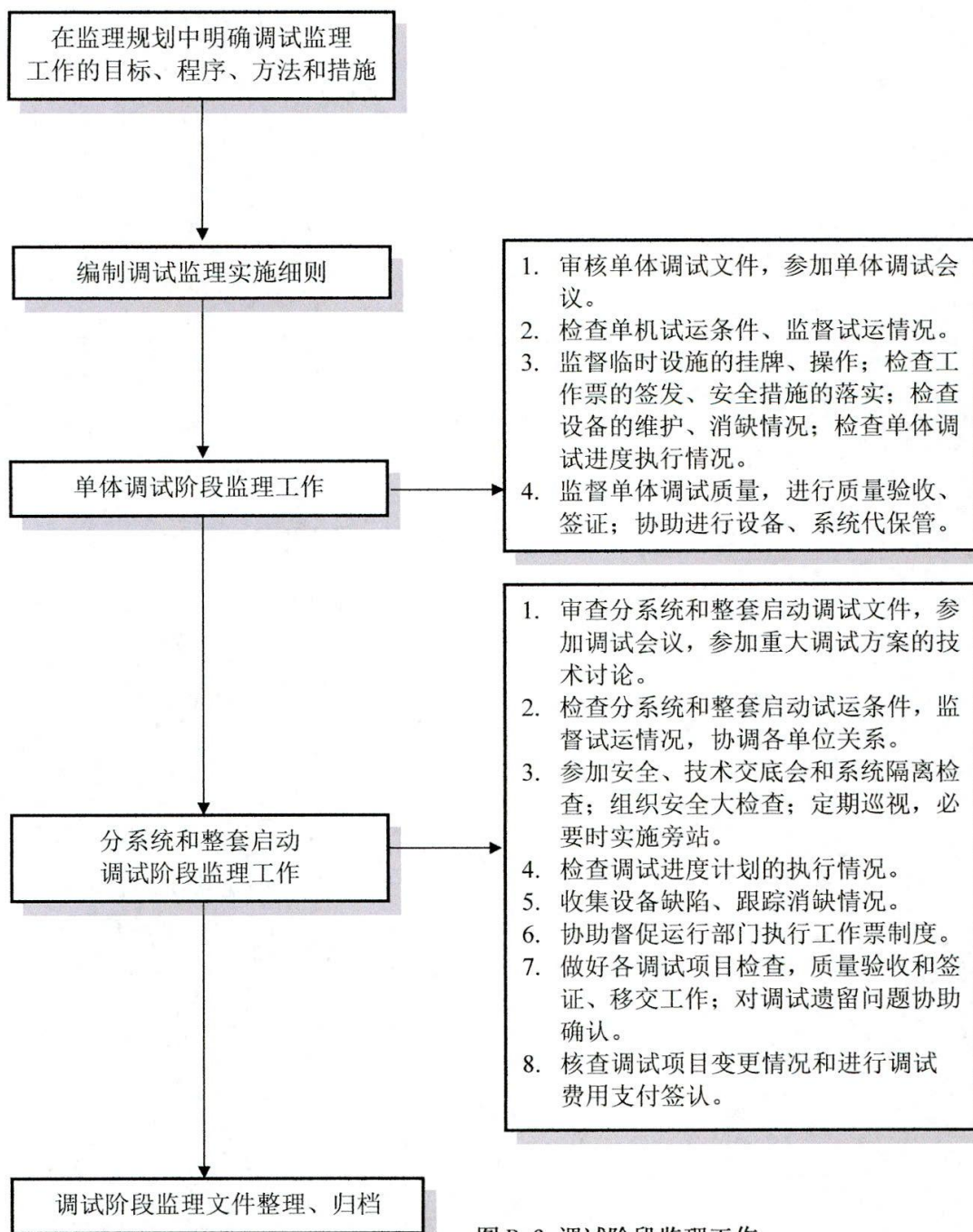
图 B.6 调试阶段监理工作
