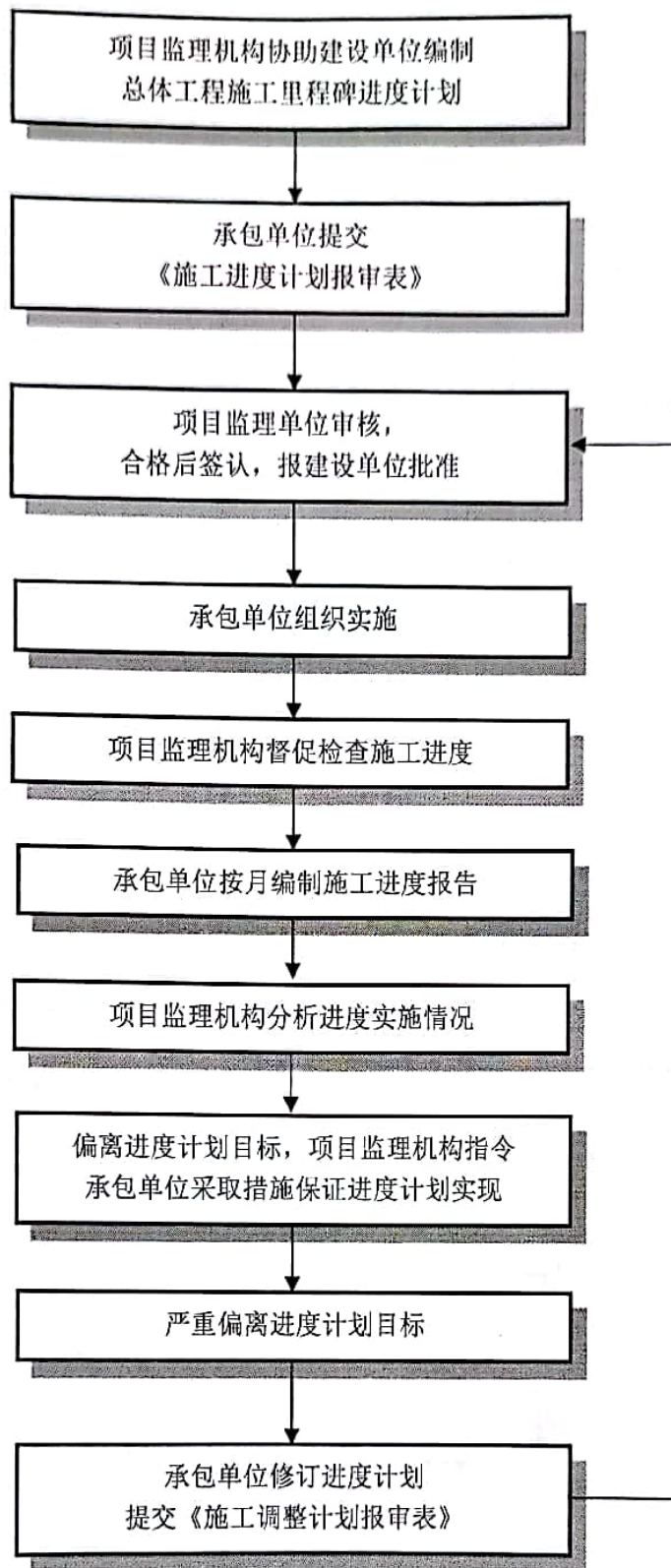
图 B.2 施工阶段工程进度监理程序框图
