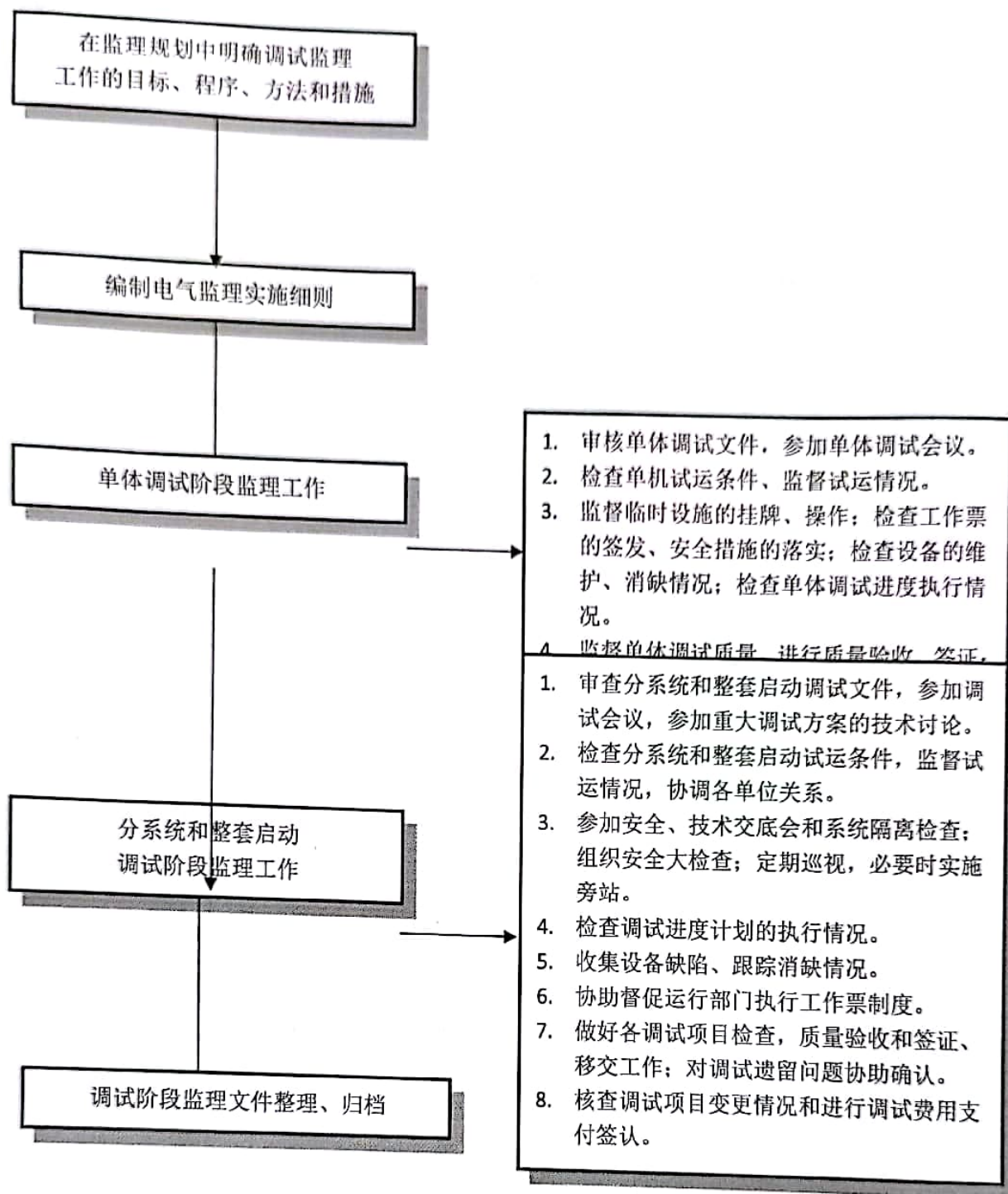
图 B.6 调试阶段监理工作程序框图
