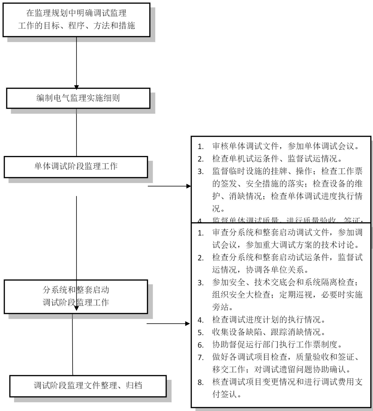
图 B.6 调试阶段监督工作程序框图
