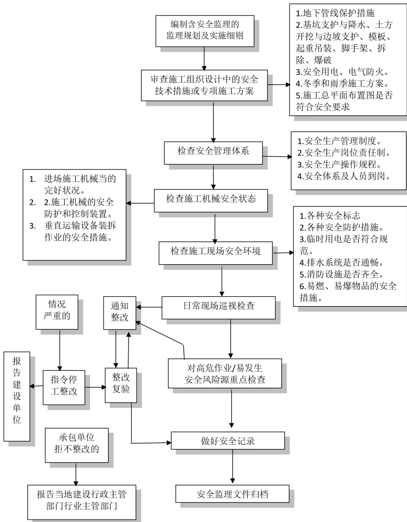
图 B.2 施工阶段工程进度监理程序框图
