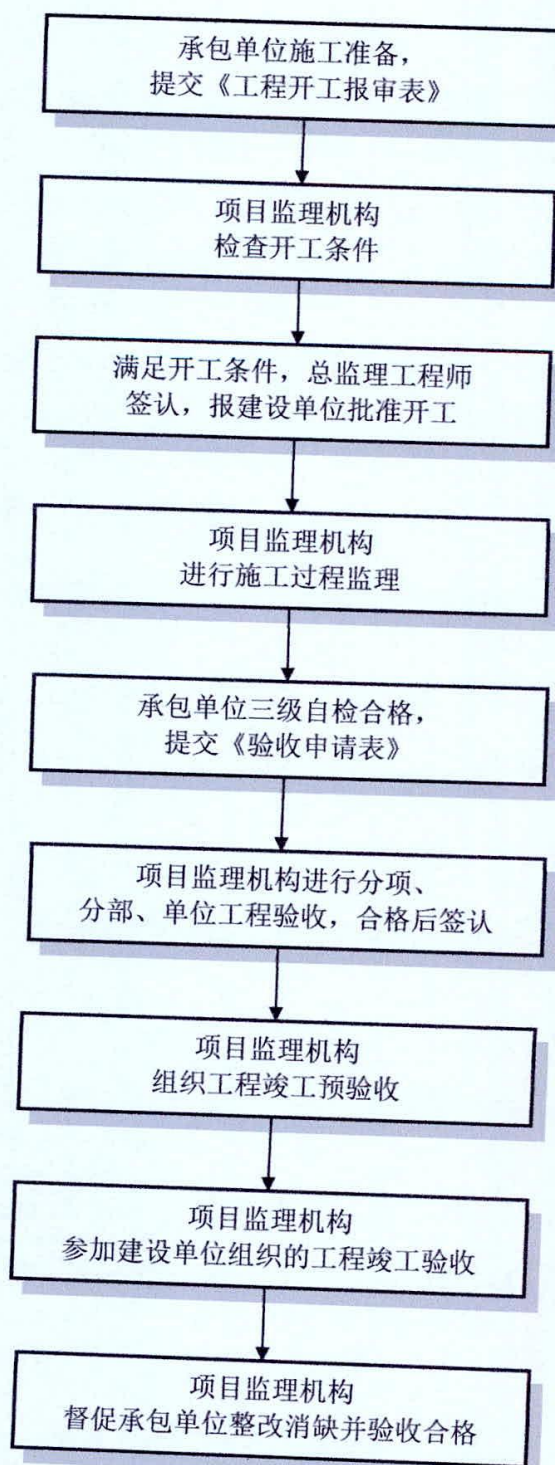
图 D 1 施工阶段工程验收程序图
