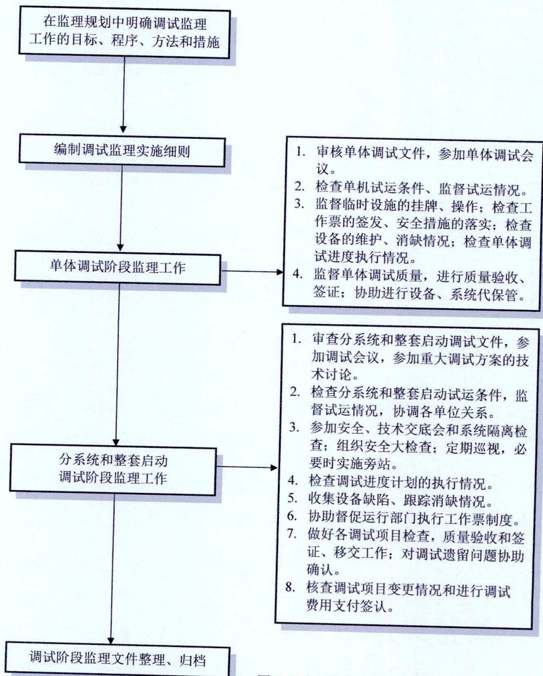
图 B.6 调试阶段监理工作
