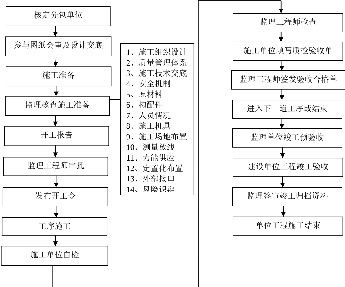
单位工程施工监理质量控制流程
