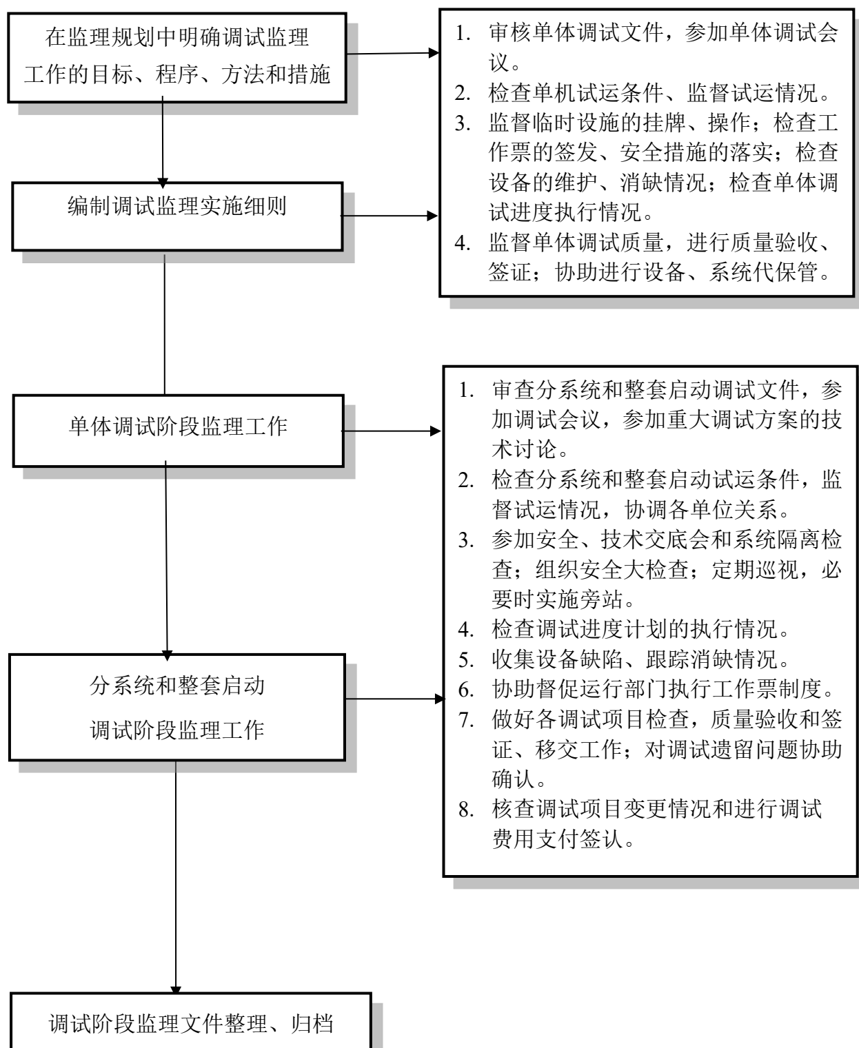
图 B.9 调试阶段监理工作程序框图
