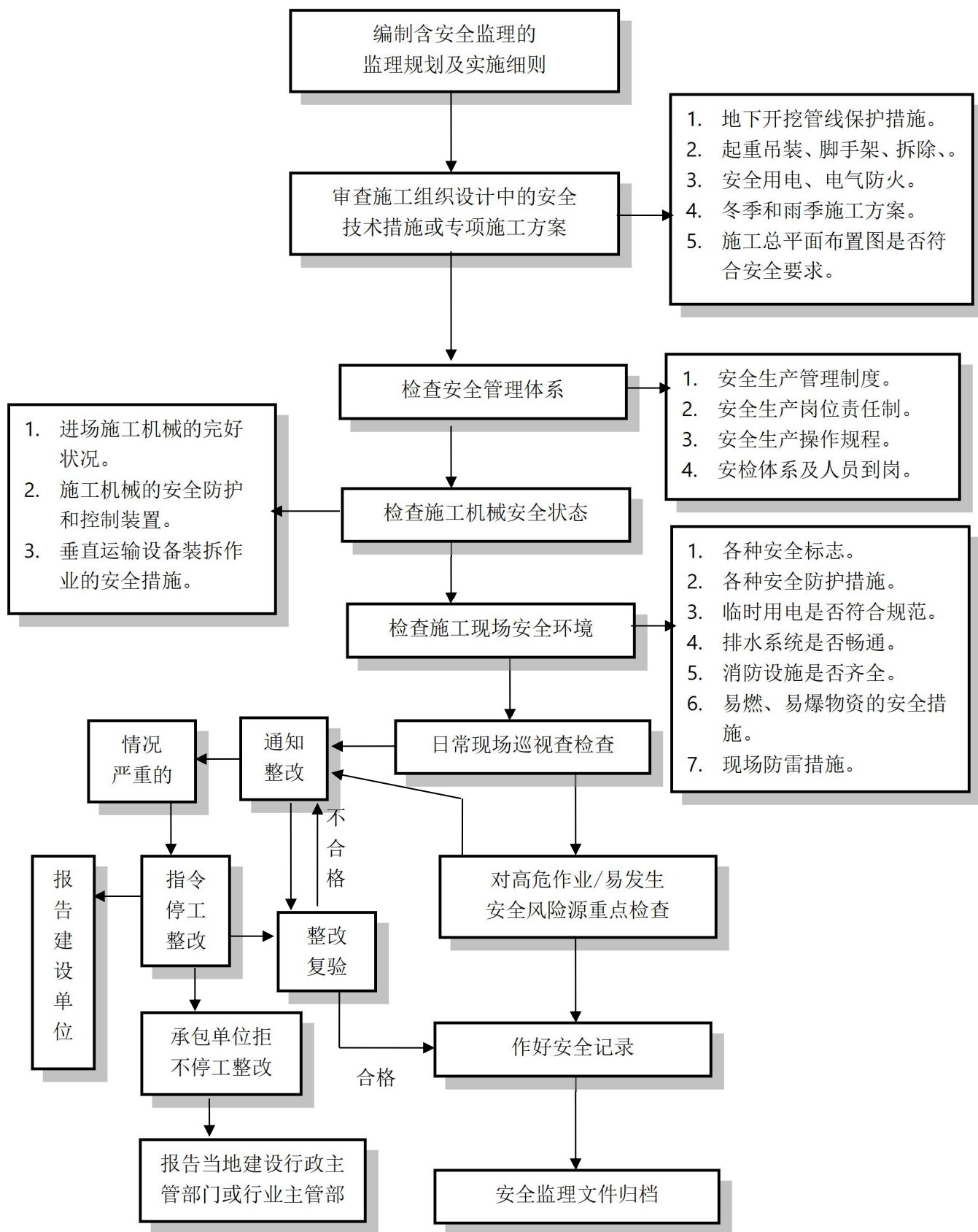
图 B.3 施工阶段工程安全监程序框图
