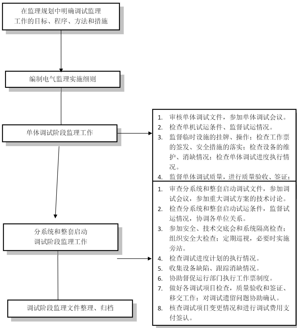
图 B.6 调试阶段监理工作程序框图
