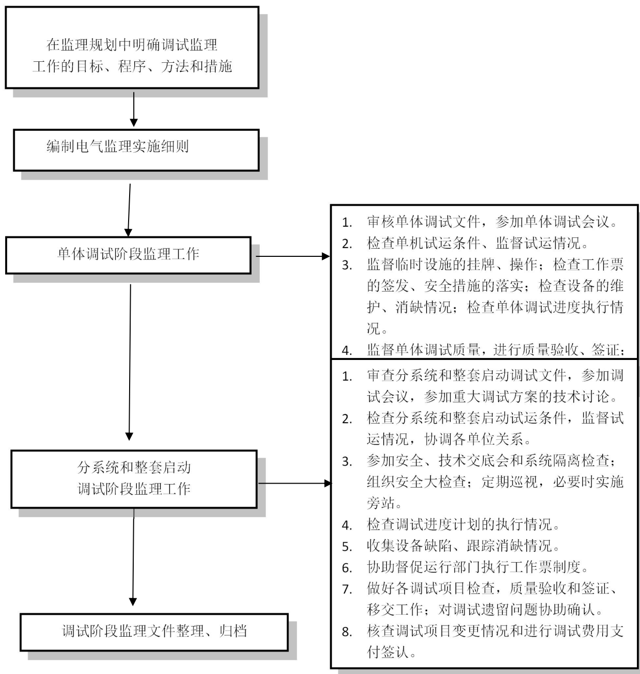
图 B.6 调试阶段监督工作程序框图
