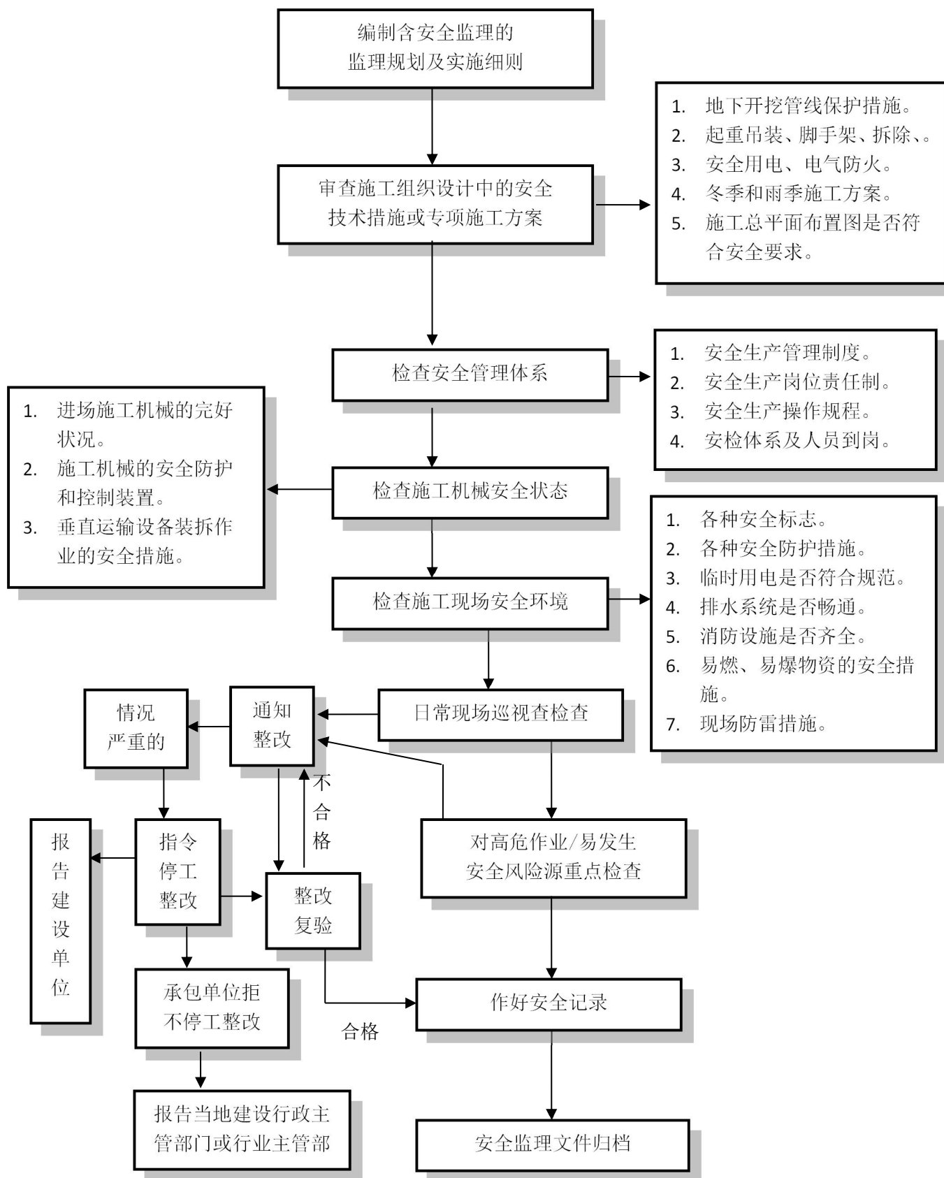
图 B.3 施工阶段工程安全监程序框图
