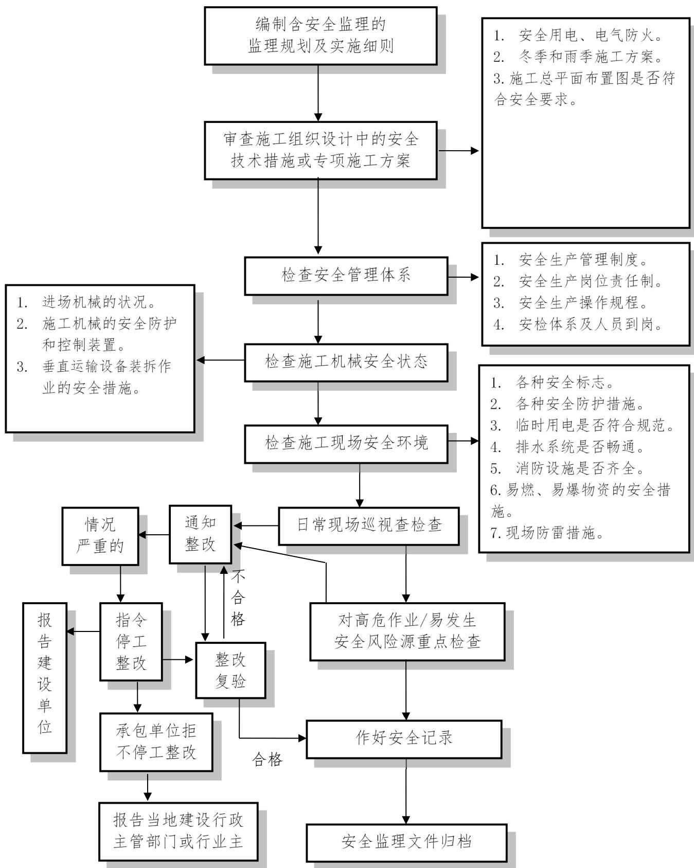
图 3 施工阶段工程安全监程序框图
