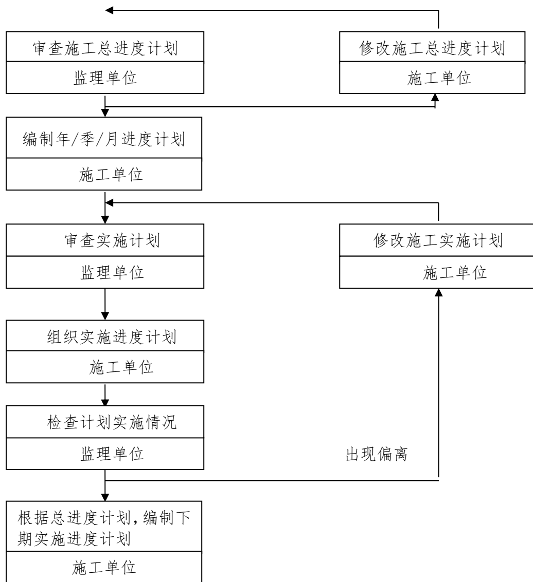
2) 施工进度计划的申报与审批程序 (流程图二)
