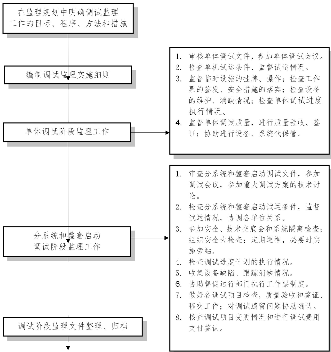
图 6 调试阶段监理工作程序框图
