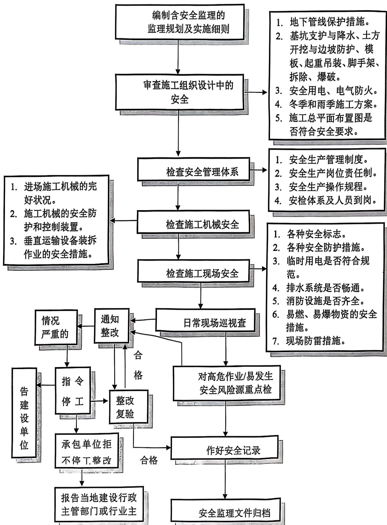
图 B.3 施工阶段工程安全监程序框图
