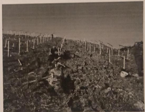
支架安装不合格照片
