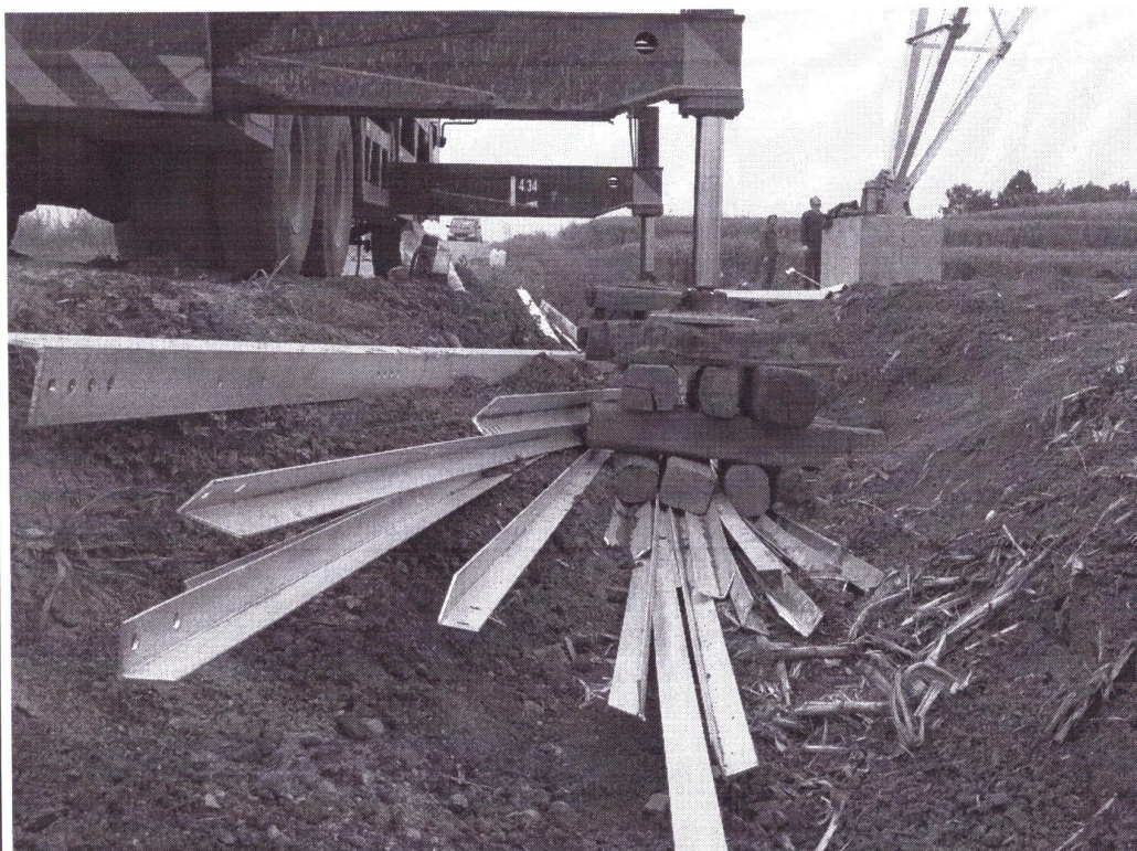
塔材被压
