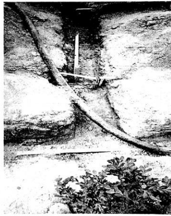
箱变接地未形成环网
