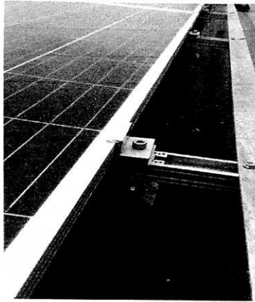
压块未安装到位
