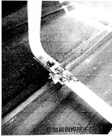
接地扁钢焊接不符合要求
