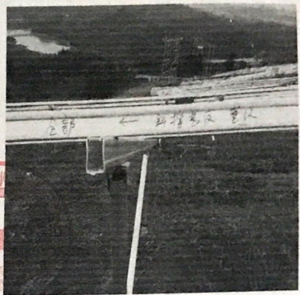
斜撑装反
