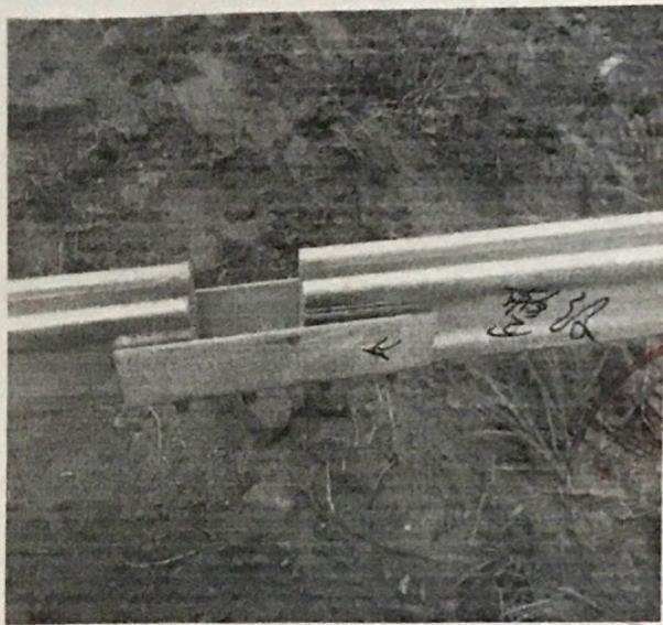
连接件空隙过大
