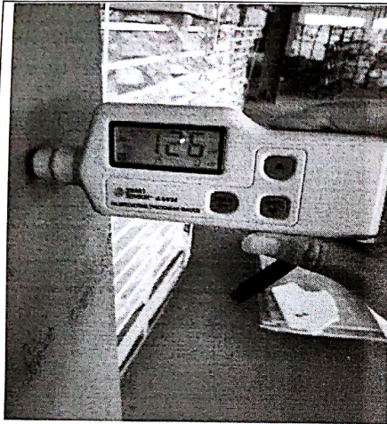
厂房防腐涂层厚度
