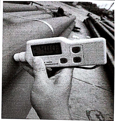
现场加固材料防腐涂层厚度
