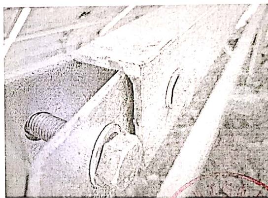
3、檩条、C型钢切口处未做防腐处理
