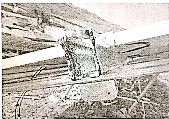
3、檩条、C型钢切口处未做防腐处理
