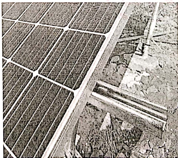
5、个别安装的组件压块缺失
