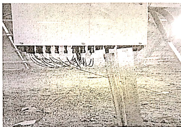
8、接地扁铁未延沟敷设；接地扁铁未焊接到位
