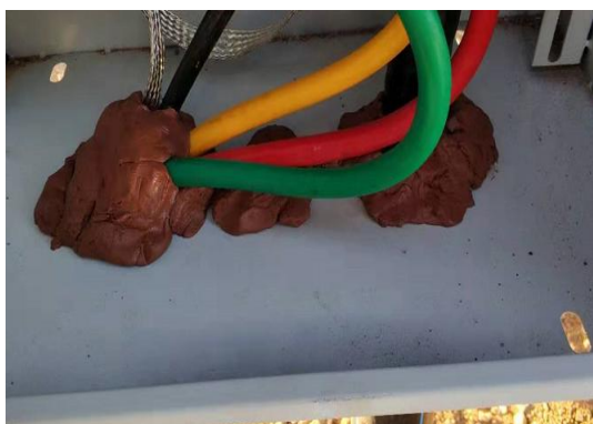
5、压块安装不合格
