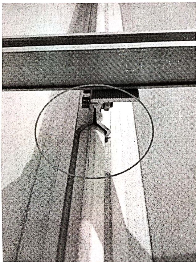
图 3：支架夹具紧固不到位
