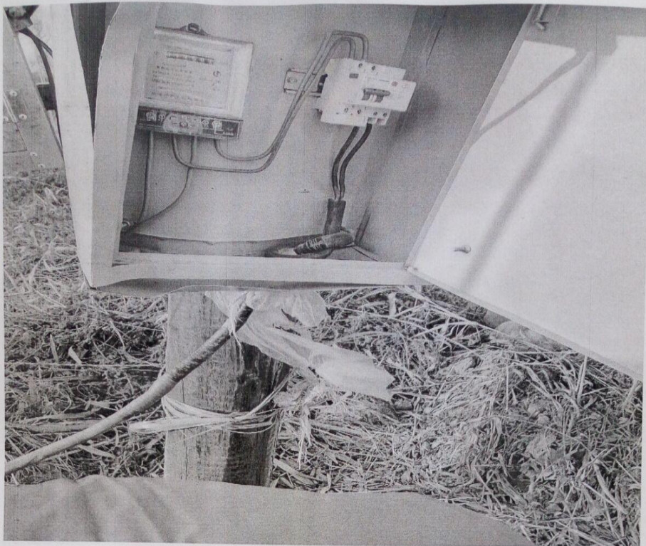
未做接地、线缆与开关连接出裸露、配电箱损坏
