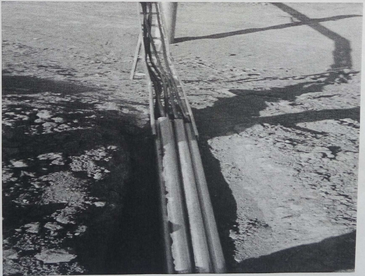
跨池埂穿线镀锌管为延伸至桥架内 整改后
