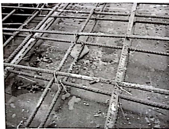
钢筋保护层
