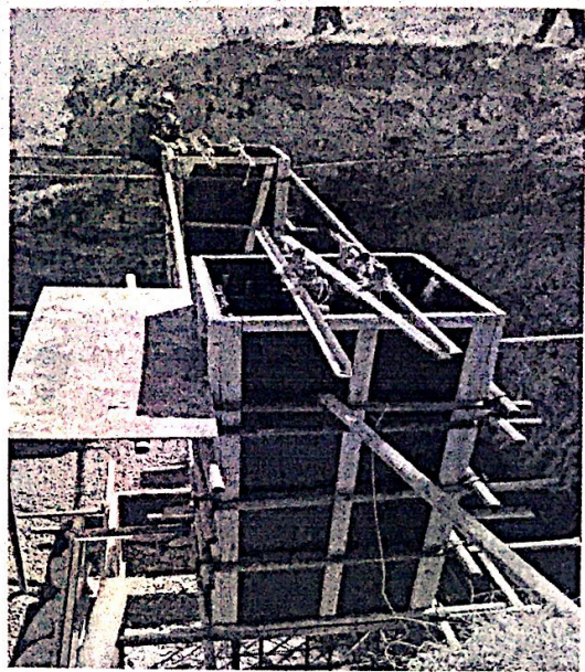
只有一个柱体安全操作平台
