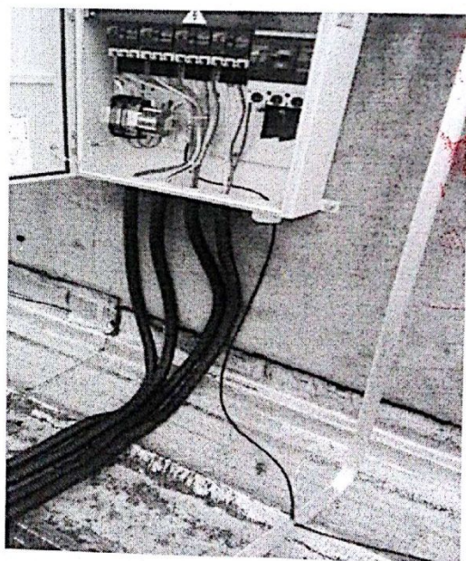
接地线不符合要求
